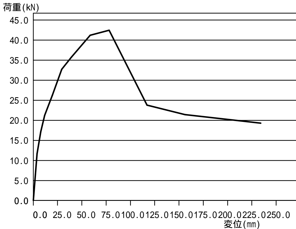
1 階 Y方向 X10' 9.100m 荷重-変形関係曲線
