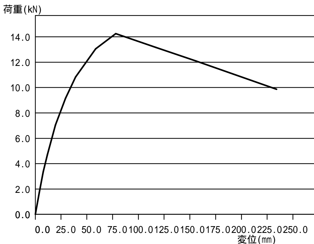
1 階 方向 Y9 7.280m 荷重-変形関係曲線
