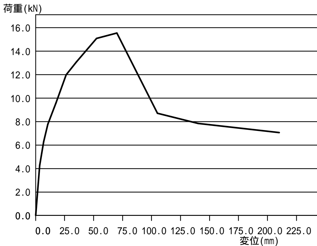
2階 Y方向 X21 18.570m 荷重-変形関係曲線
