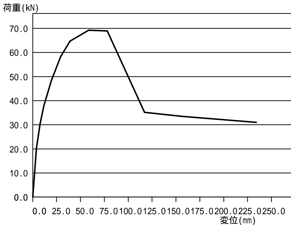
1階 Y方向 X35 31.310m 荷重-変形関係曲線
