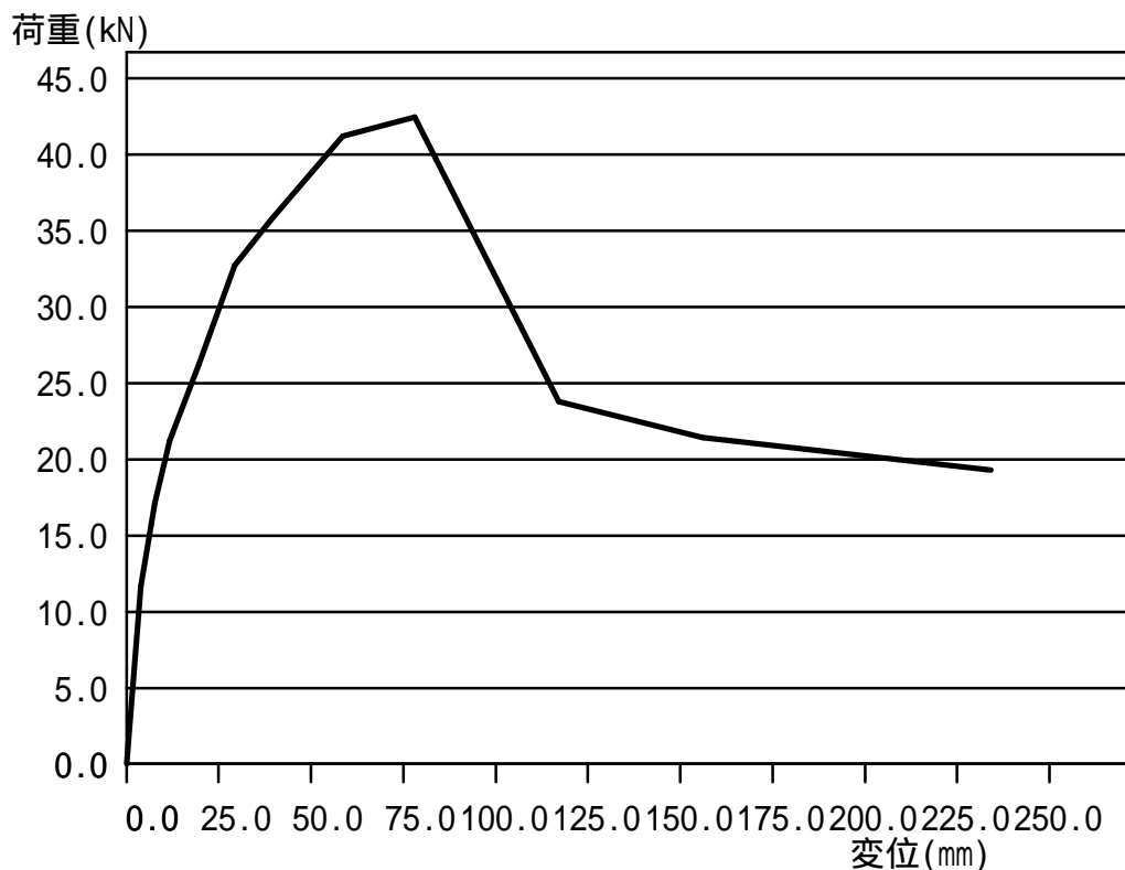
1階 Y方向 X25 22.210m 荷重-変形関係曲線
