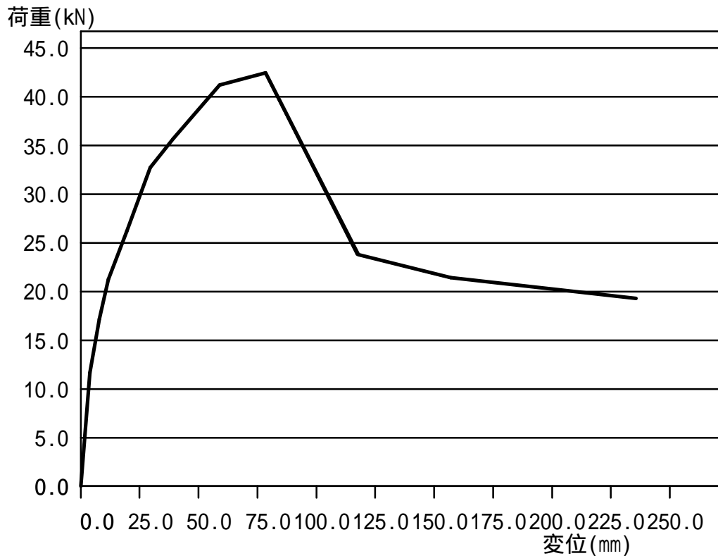
1 階 Y 方向 X21 18.570m 荷重-変形関係曲線(ねじれ補正後 補正值= 0.9934)
