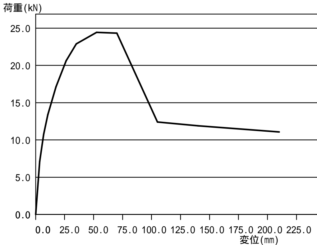
2 階 Y方向 X35 31.310m 荷重-変形関係曲線
