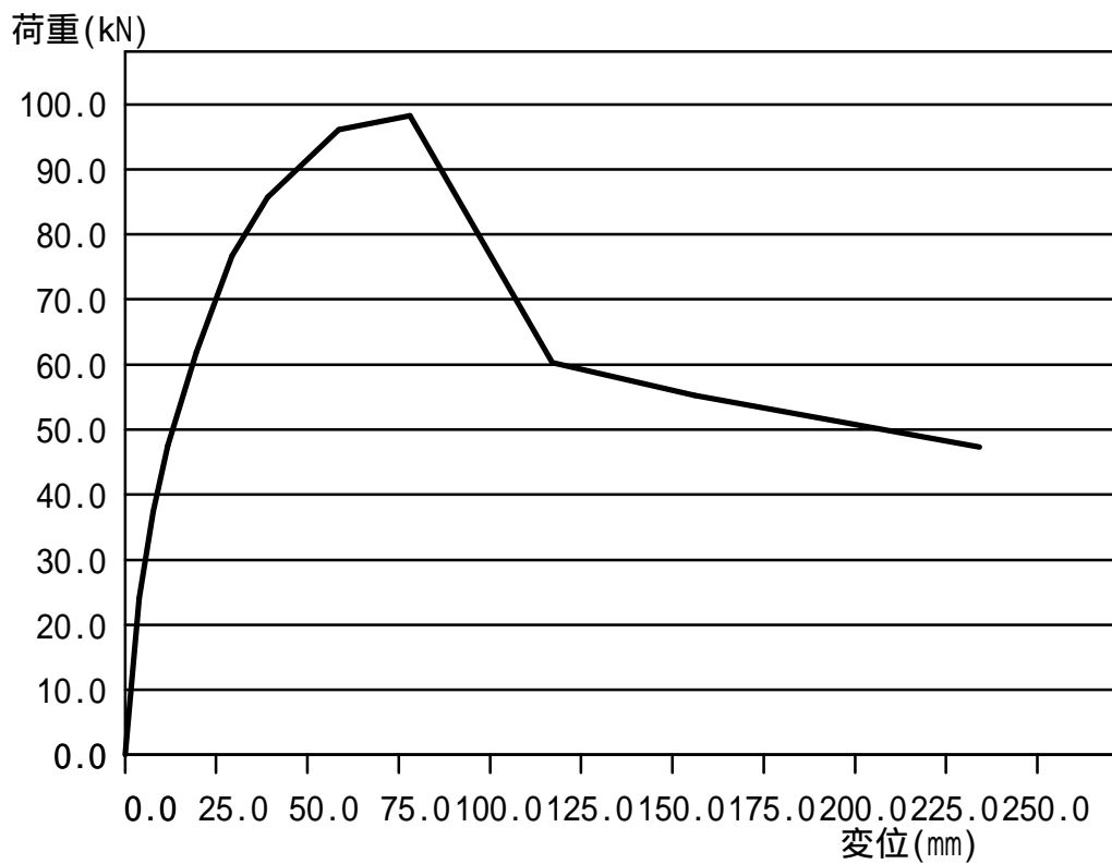
1 階 方向 Y1 0.000m 荷重-変形関係曲線
