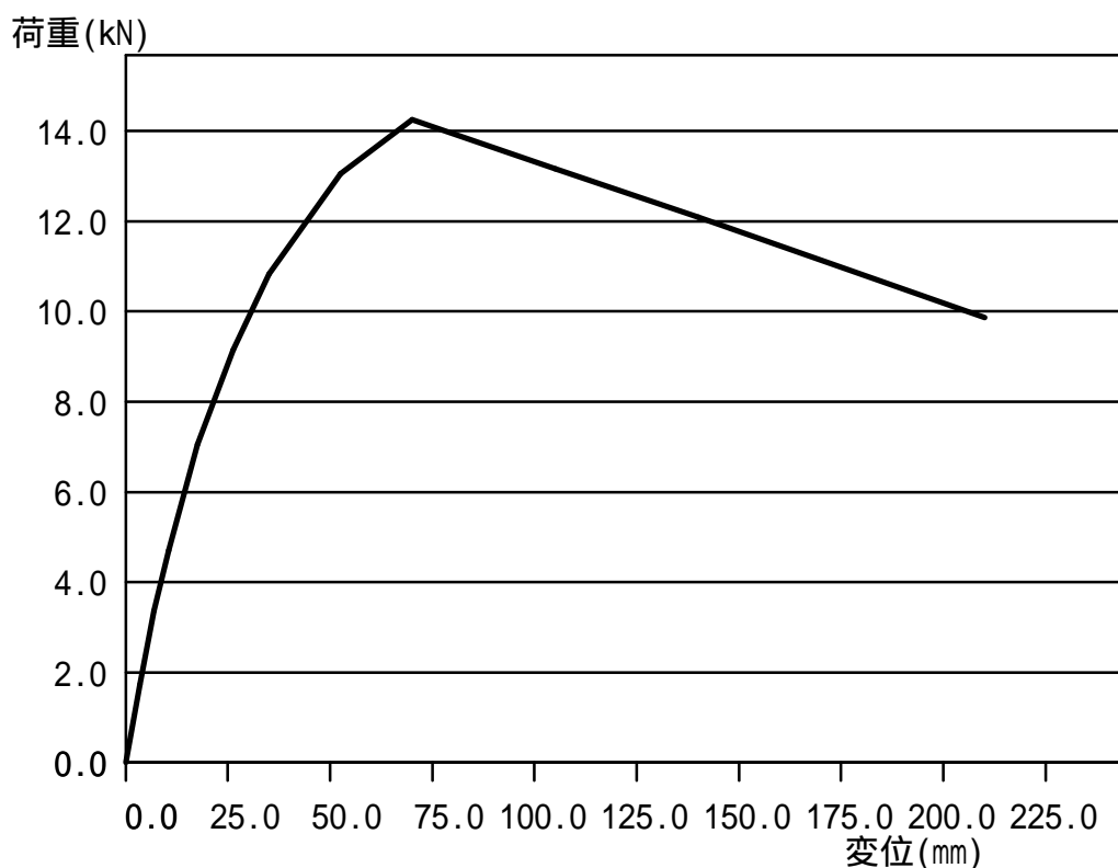
2 階 方向 Y9 7.280m 荷重-変形関係曲線
