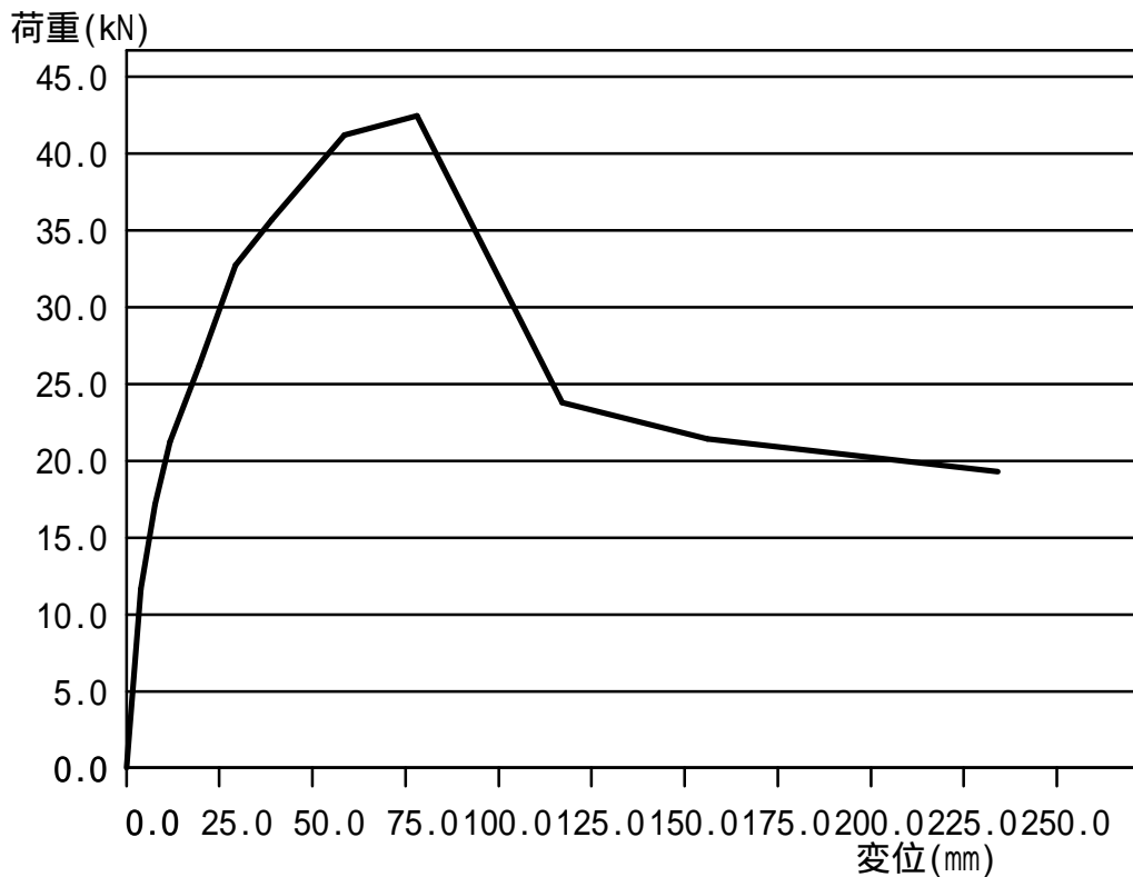
1 階 Y方向 X11 9.470m 荷重-変形関係曲線
