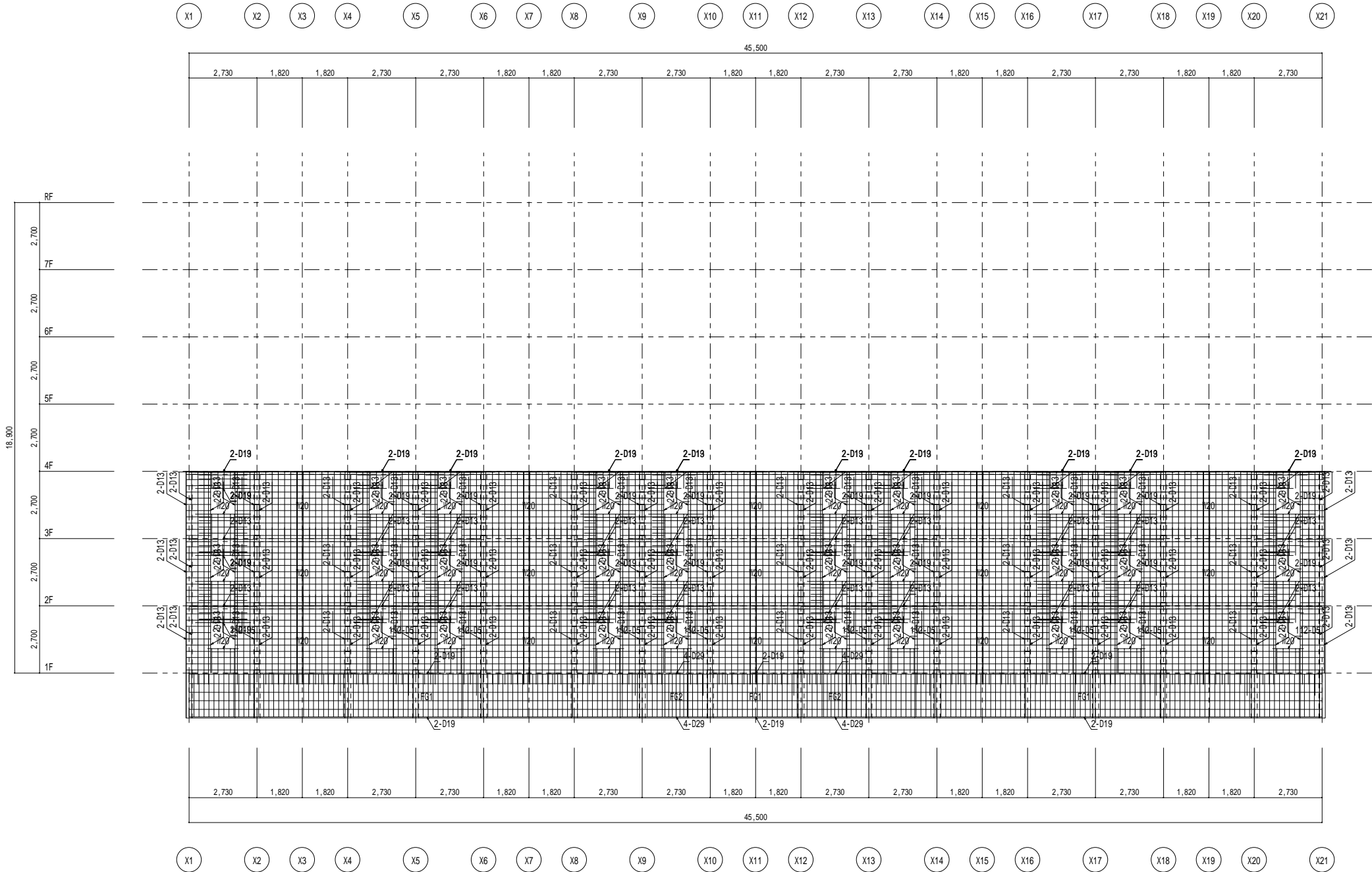
Y4通り架構詳細図 1/100
