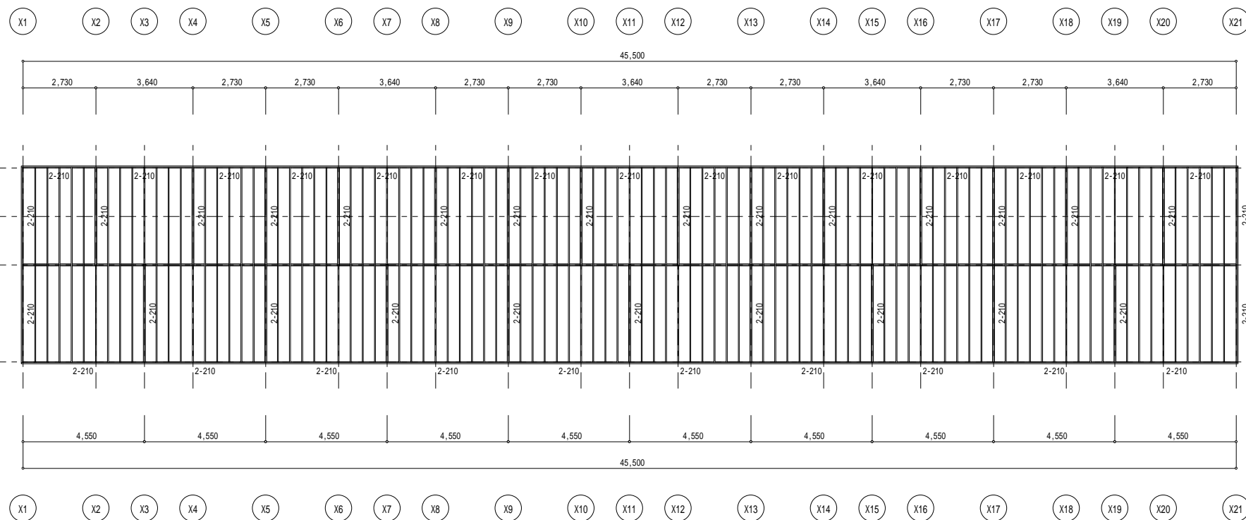
5F階床伏図 1/100
