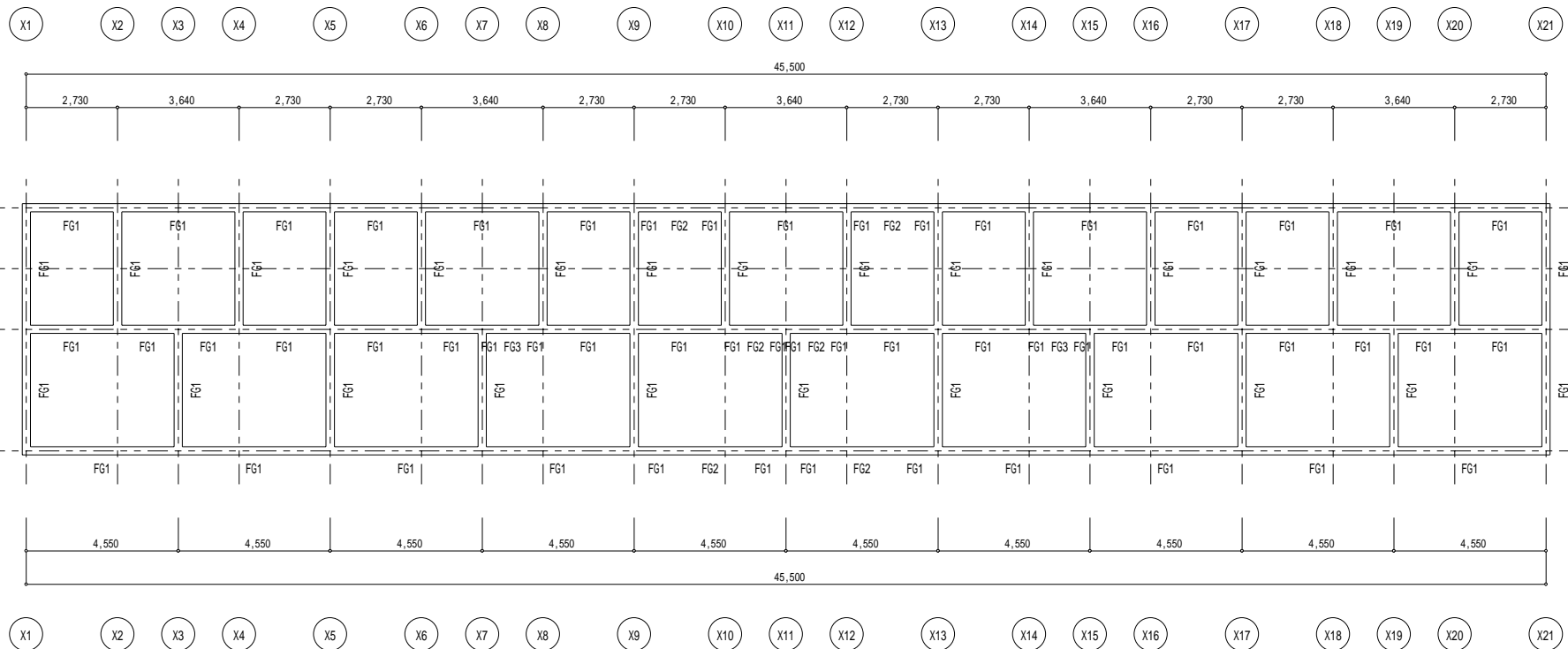
F階伏図 1/100
