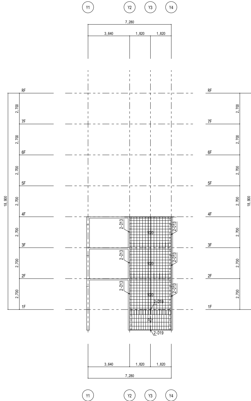
X8通り架構詳細図 1/100
