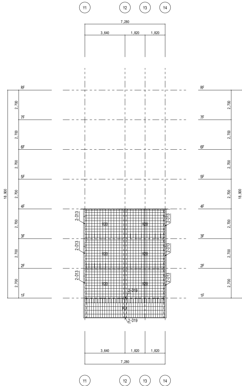
X13通り架構詳細図 1/100
