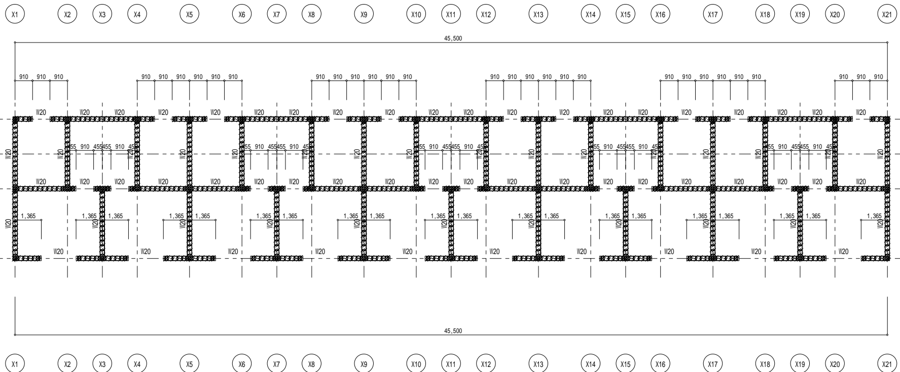
3F階平面詳細図 1/100
