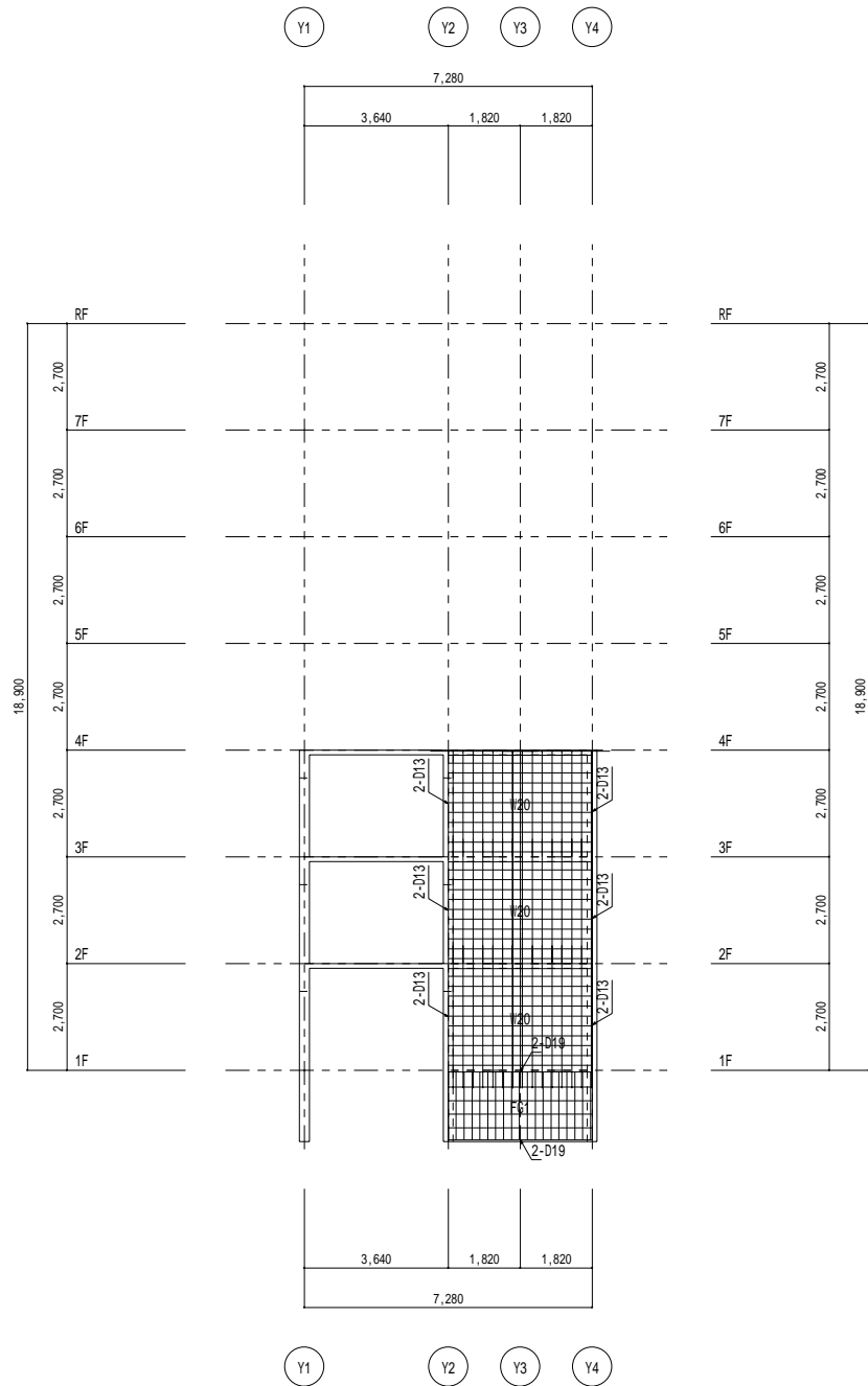
X6通り架構詳細図 1/100
