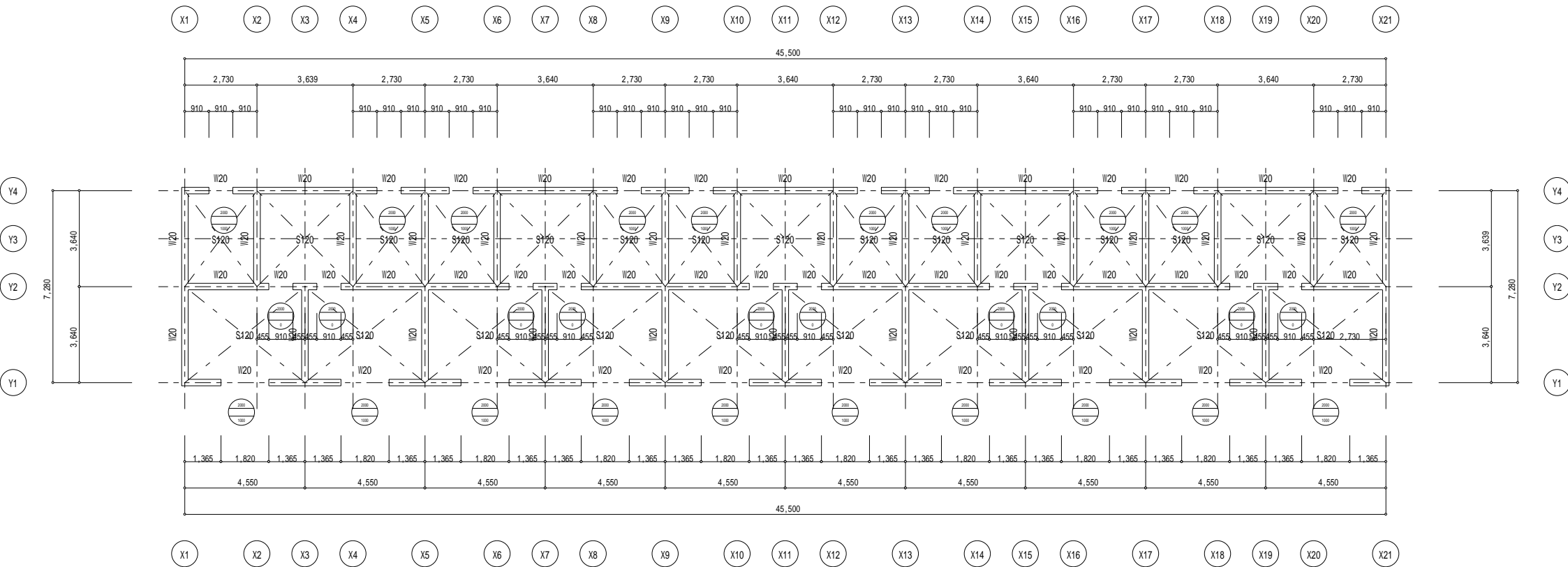
1F階伏図 1/100
