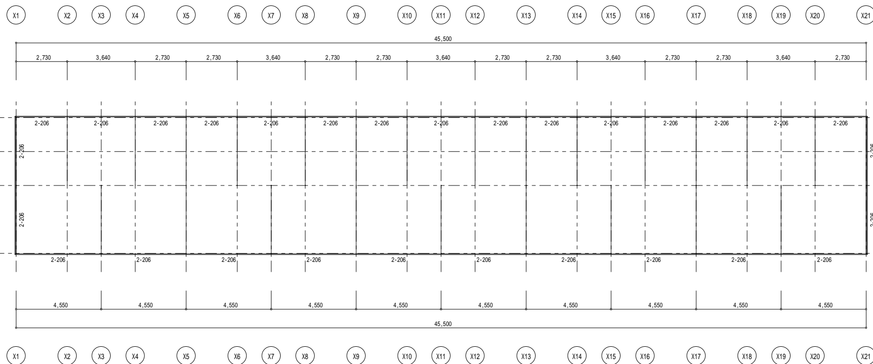
7F階床伏図 1/100
