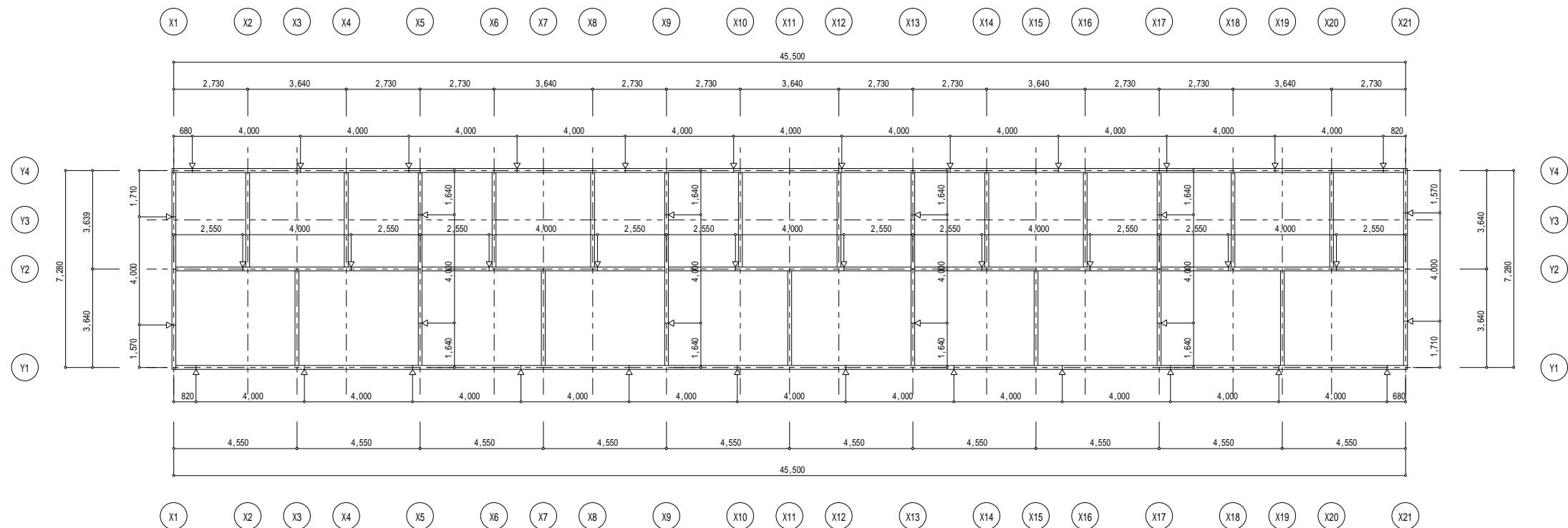
土台伏图 1/100
