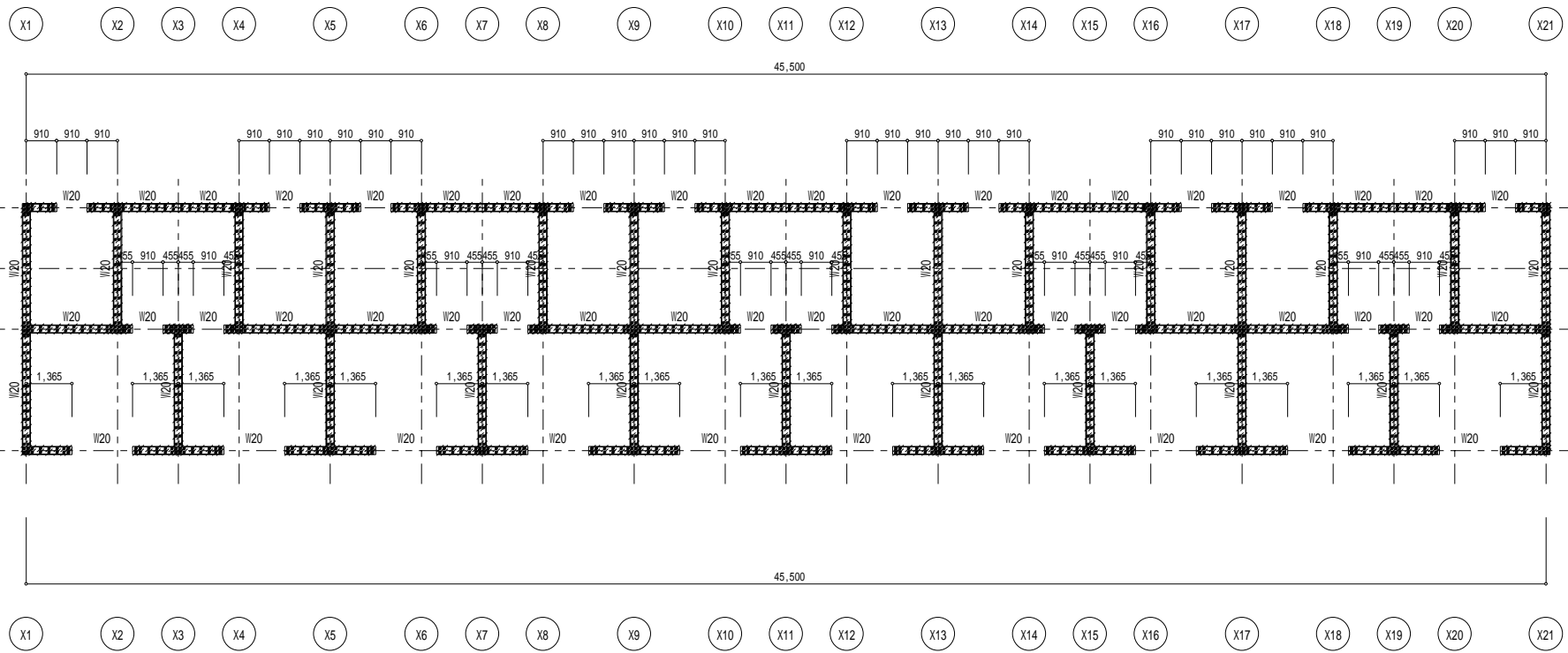
1F階平面詳細図 1/100
