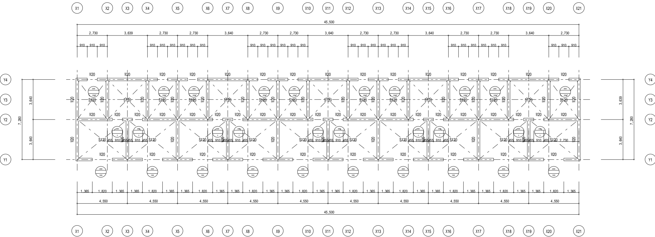
3F階伏図 1/100
