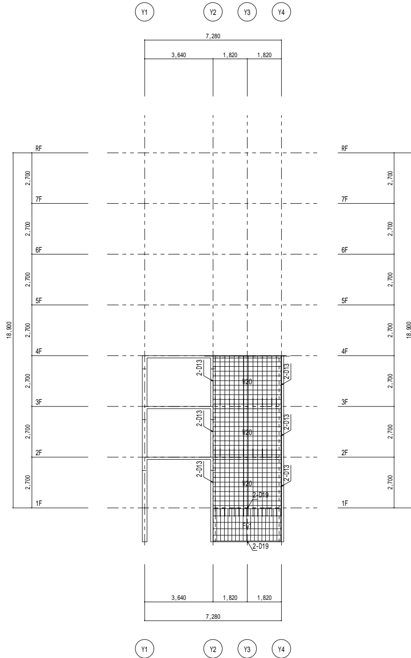
X2通り架構詳細図 1/100
