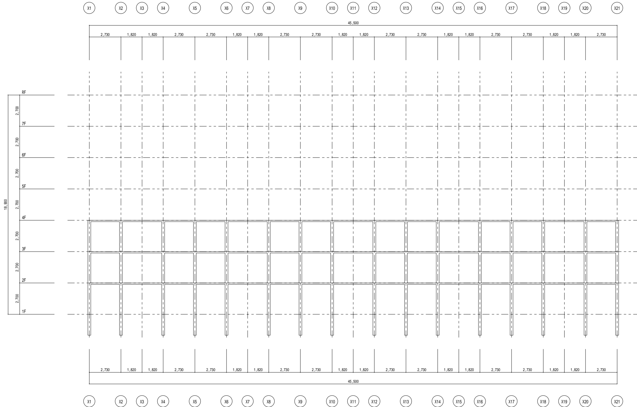
Y3通り架構詳細図 1/100
