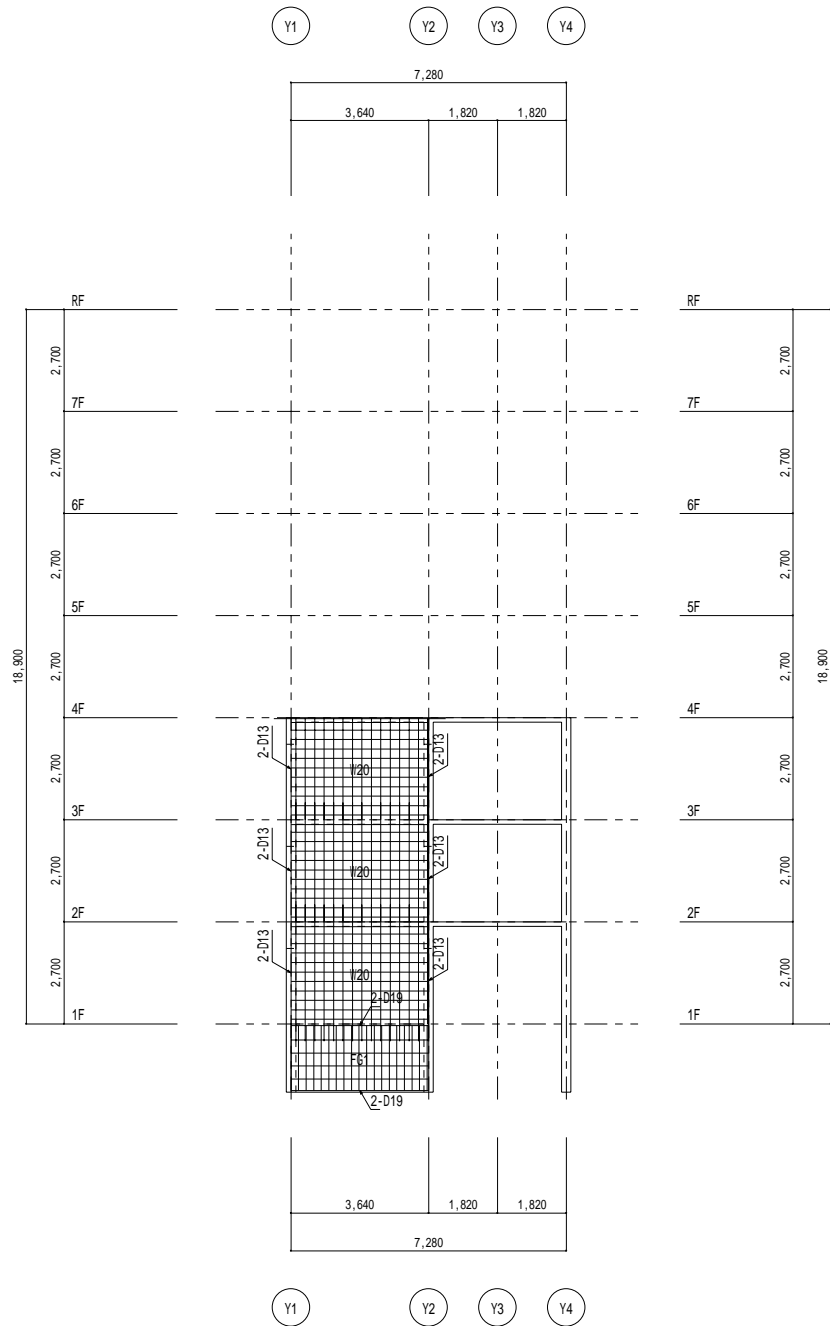
X19通り架構詳細図 1/100
