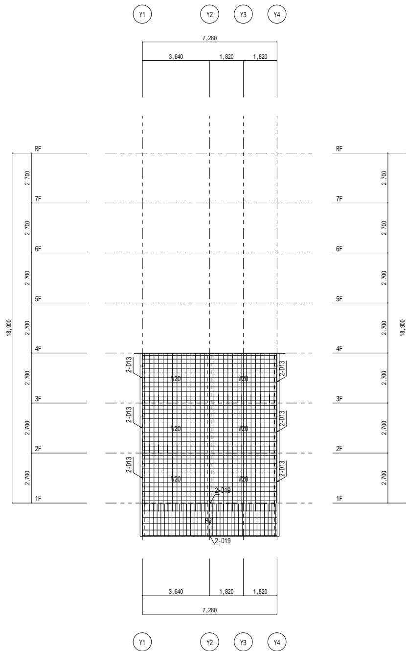
X17通り架構詳細図 1/100
