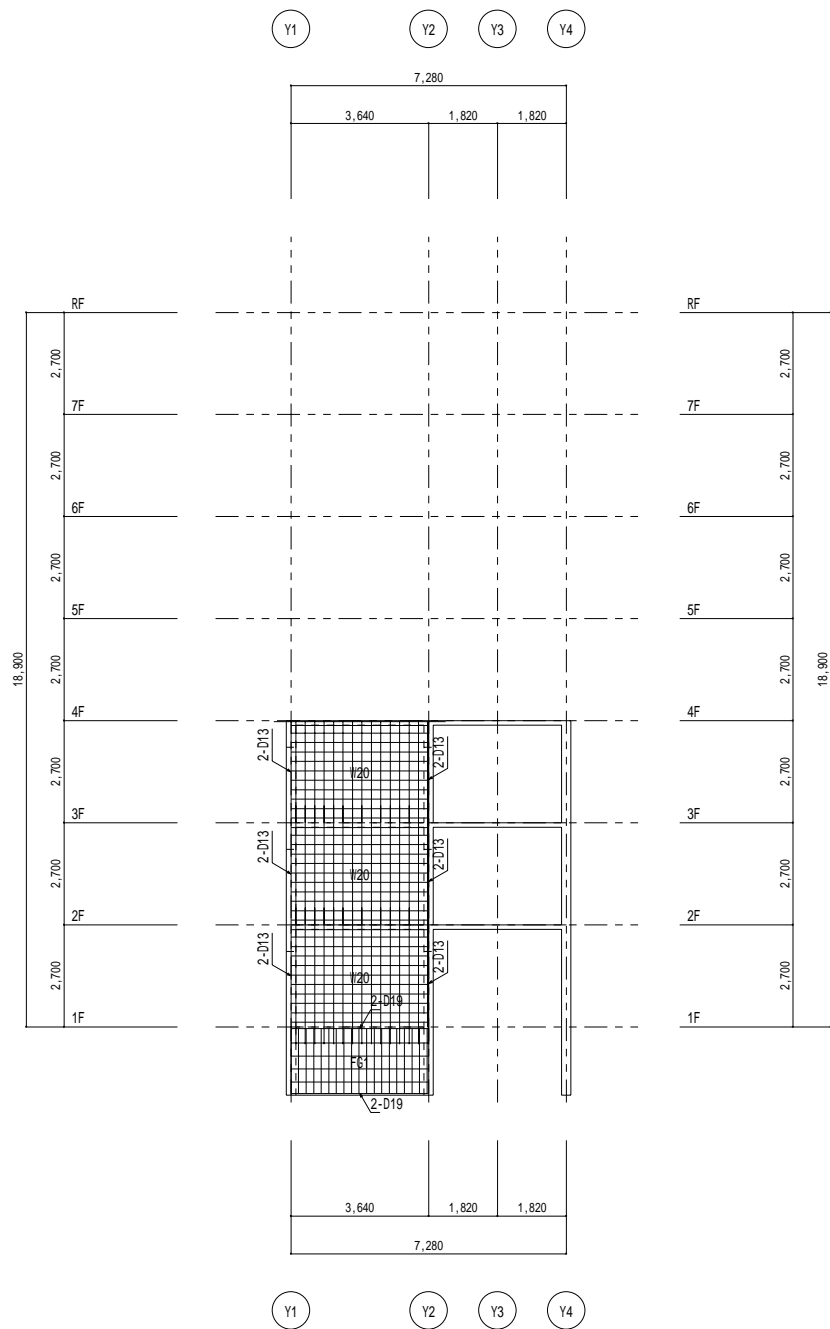
X7通り架構詳細図 1/100
