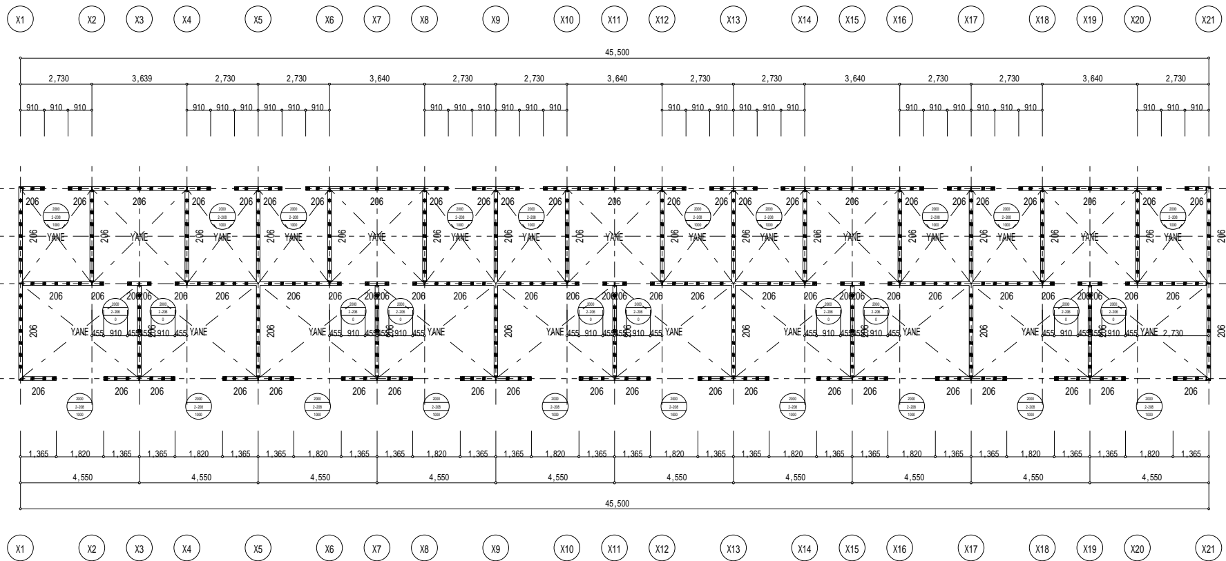
7F階たて枠伏図 1/100
