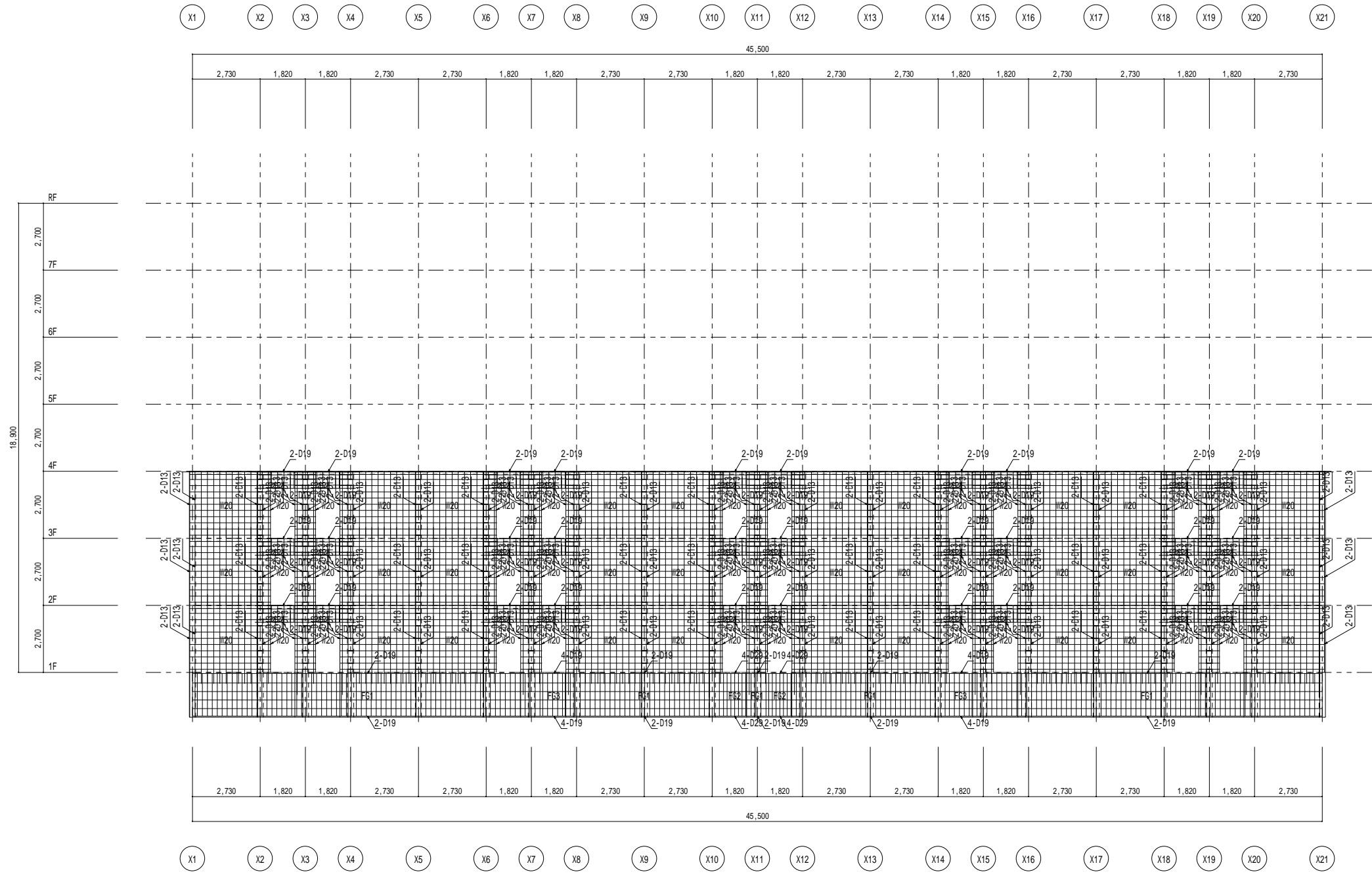
Y2通り架構詳細図 1/100
