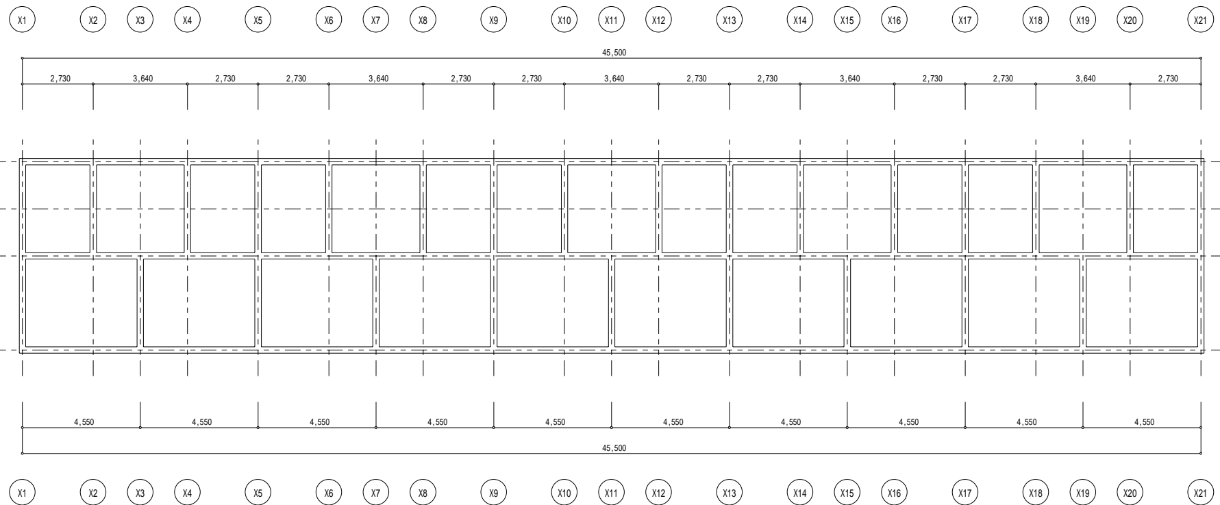
基礎伏図 1/100
