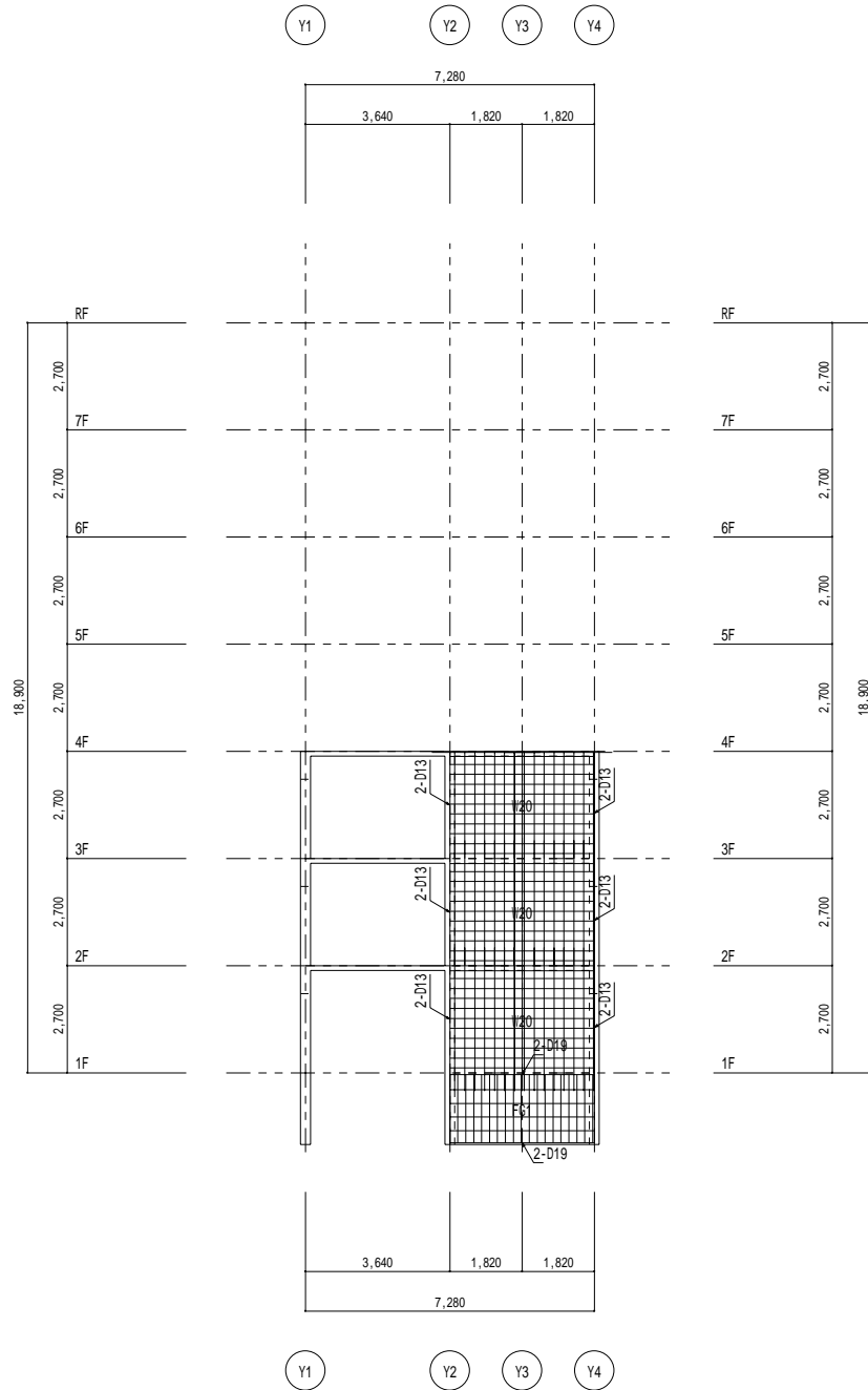
X4通り架構詳細図 1/100
