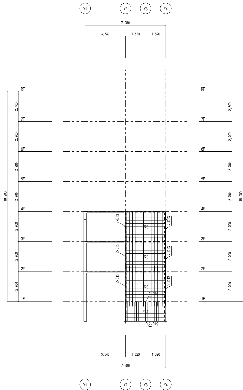
X16通り架構詳細図 1/100
