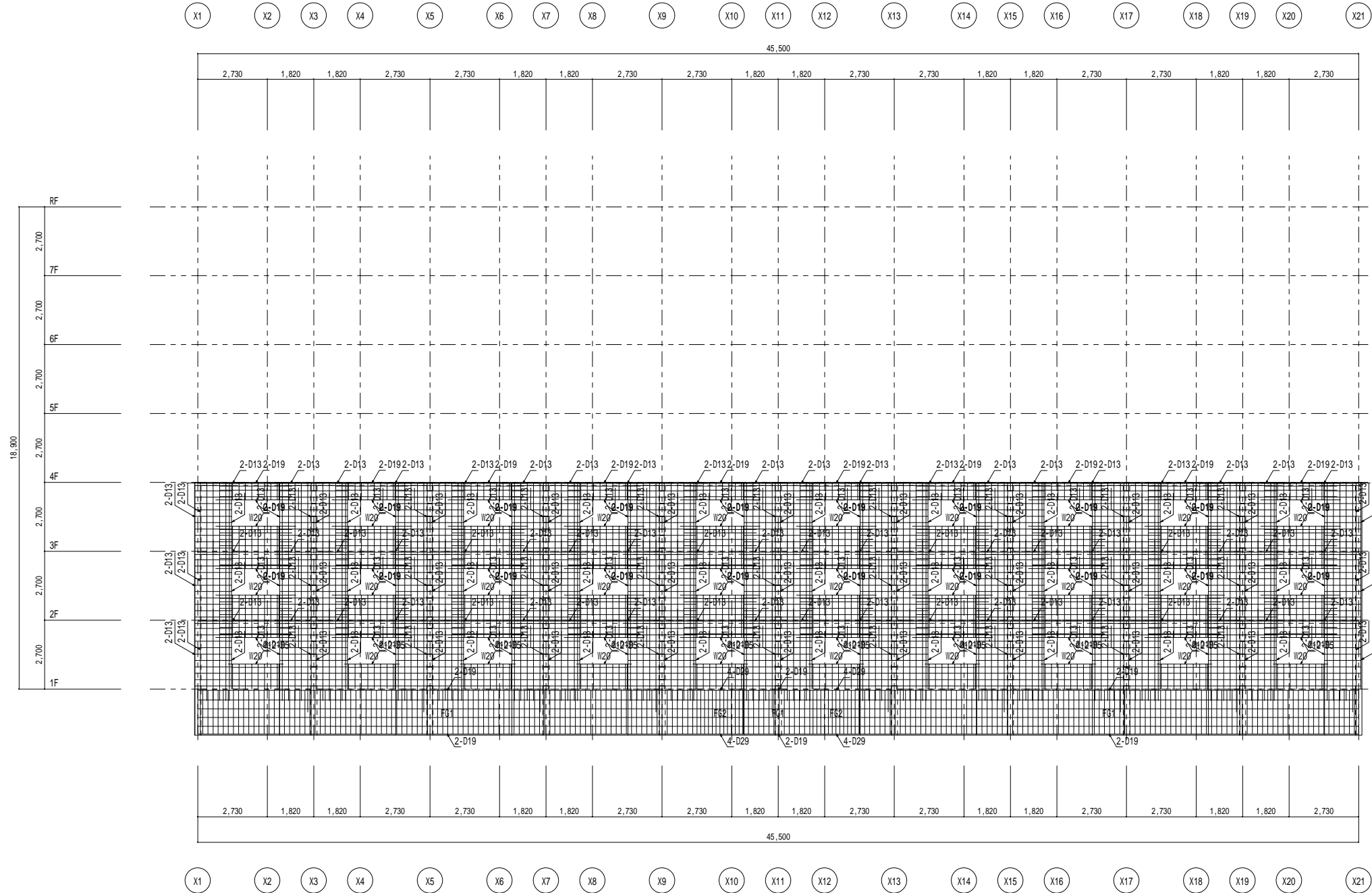
Y1通り架構詳細図 1/100
