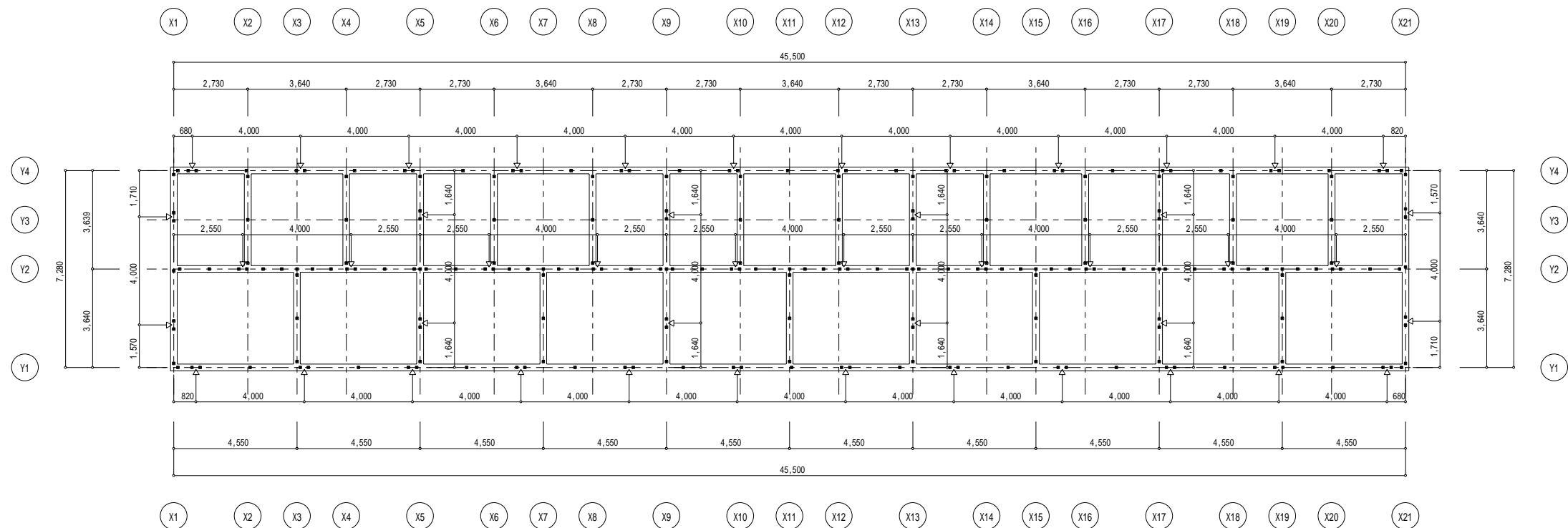
アンカー伏図 1/100
