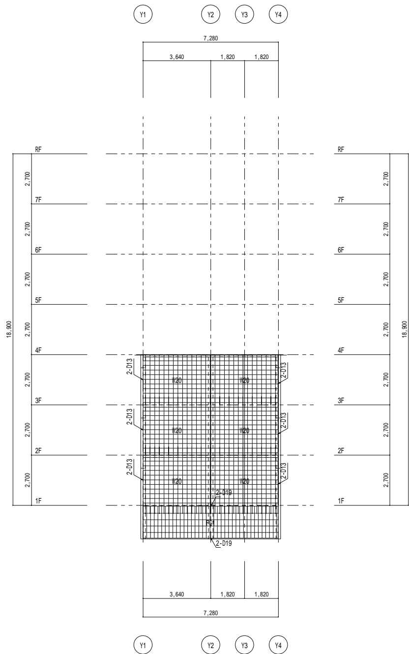
X1通り架構詳細図 1/100
