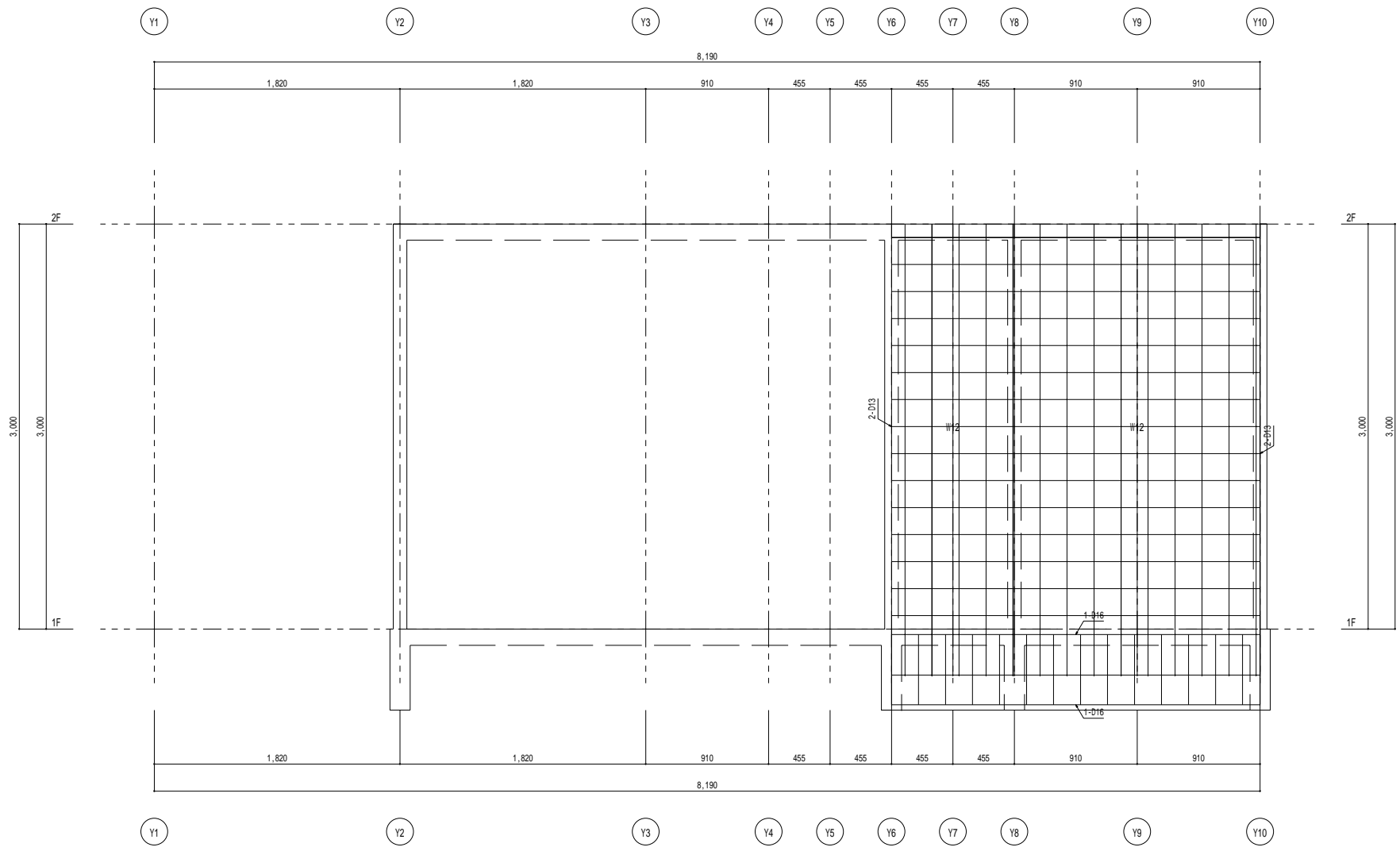
X 2 通り 架構 詳細 図 1 / 2 0
