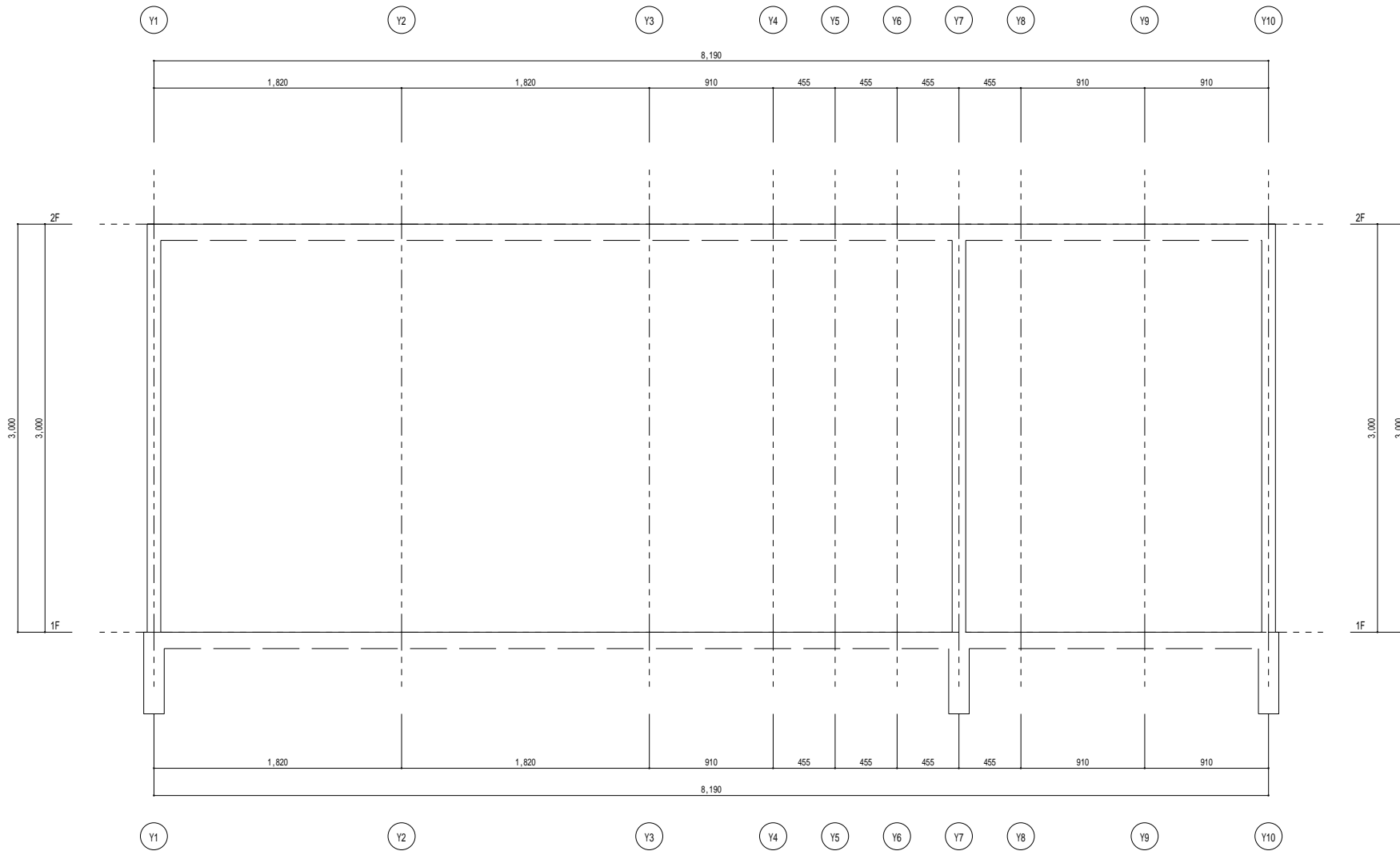
X 1 0 通リ架構詳細図 1 / 2 0
