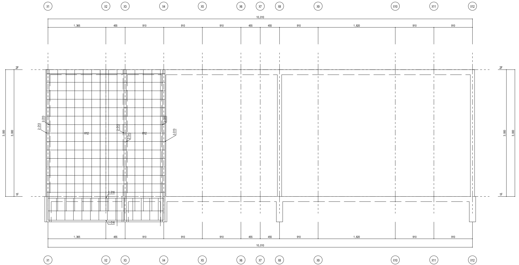
Y 2 通り架構詳細図 1 / 2 0
