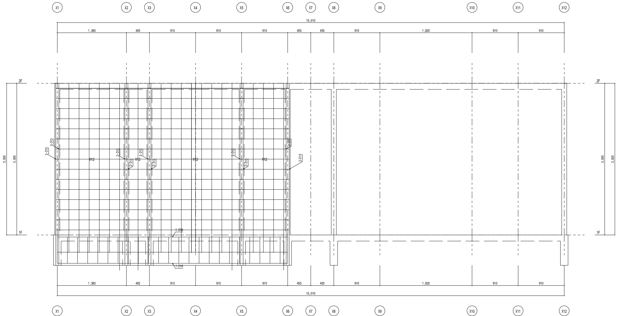
Y6 通り架構詳細図 1 / 2 0
