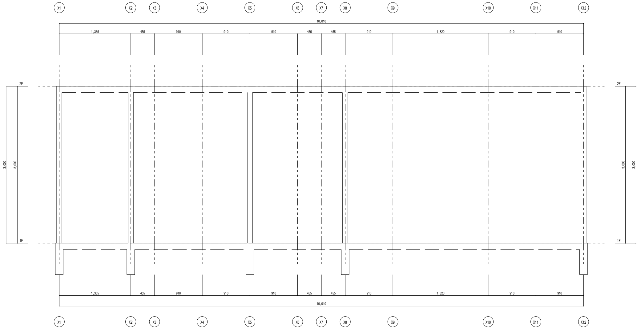
Y9通り架構詳細図 1 / 20
