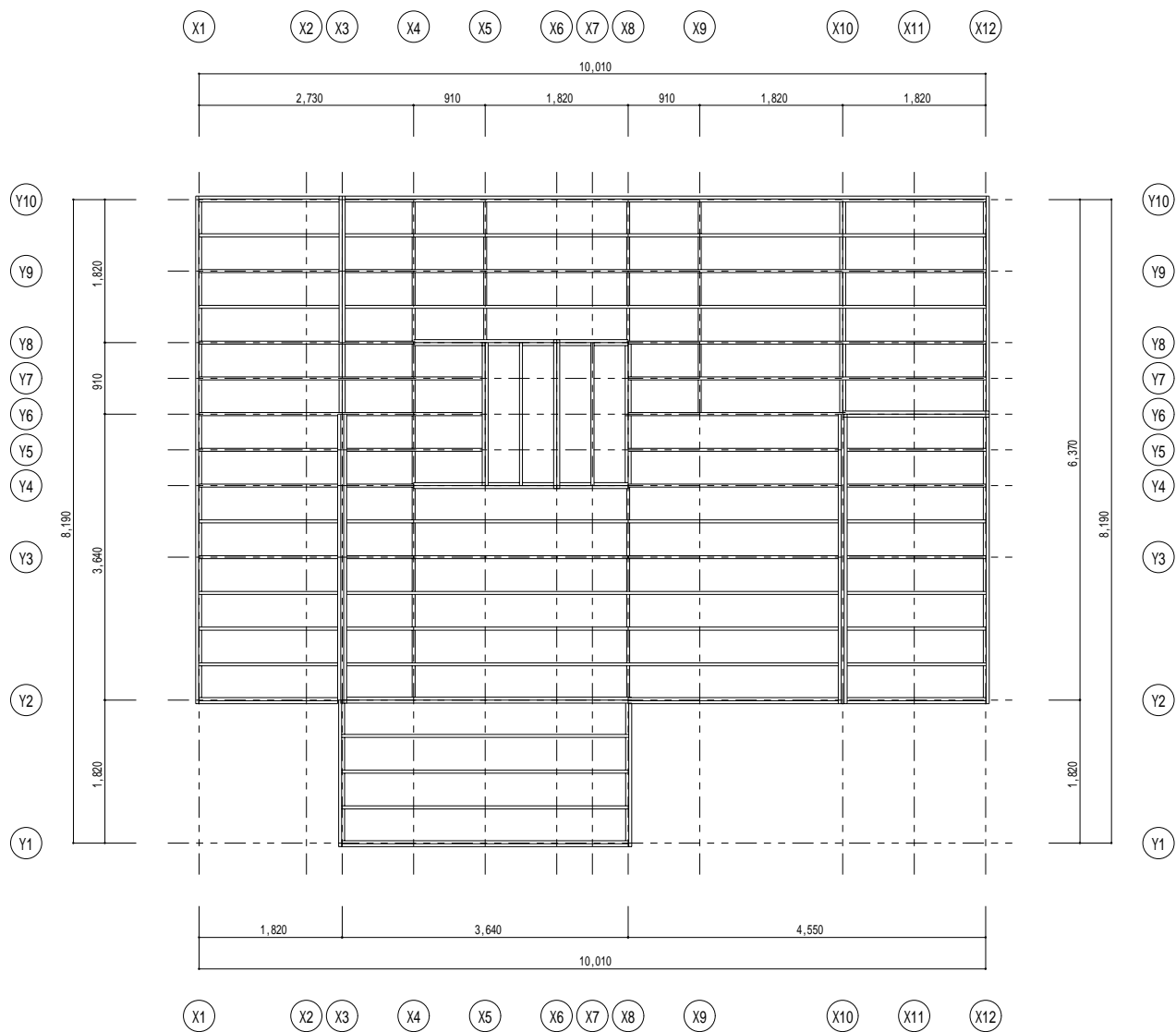
2F階床伏図 1/40
