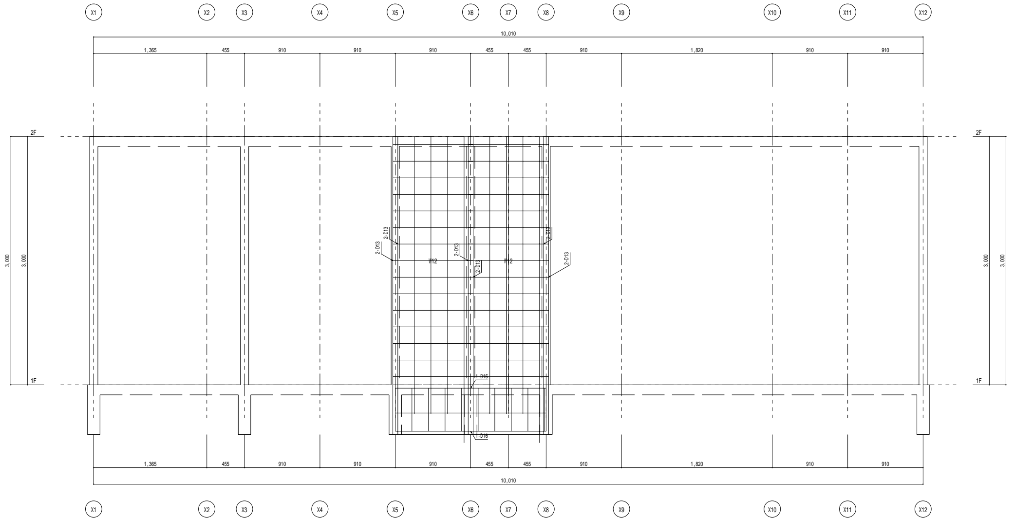
Y4 通り架構詳細図 1 / 2 0
