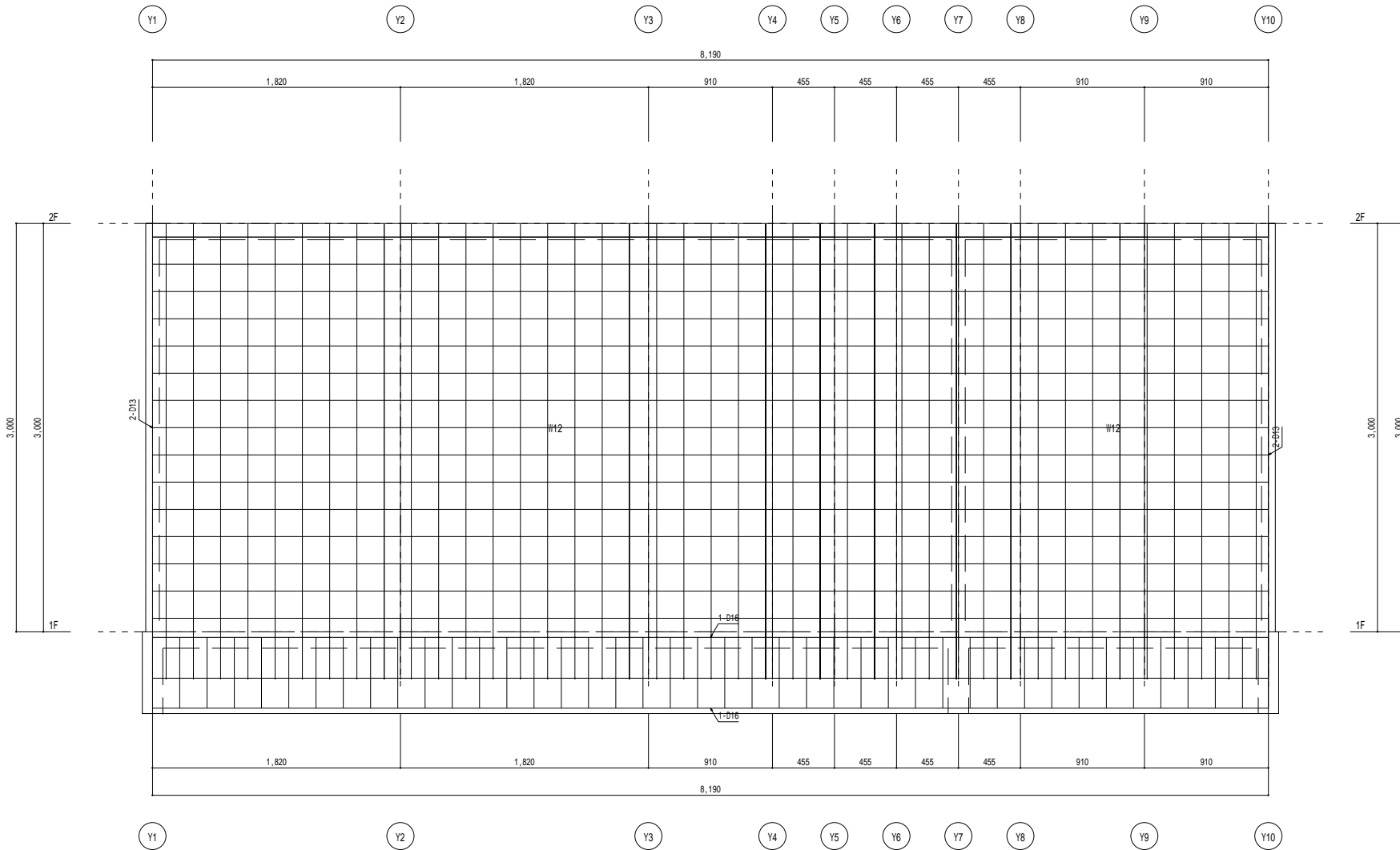
X 1.2 通り架構詳細図 1 / 20
