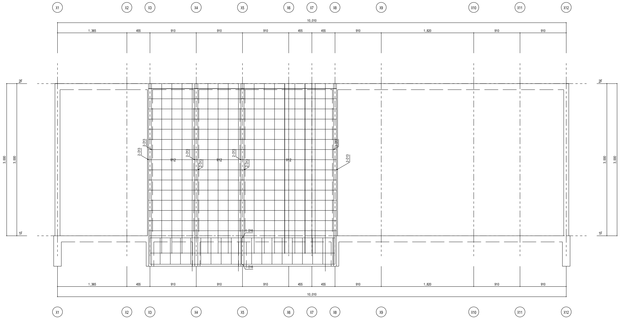
Y3通り架構詳細図 1 / 20
