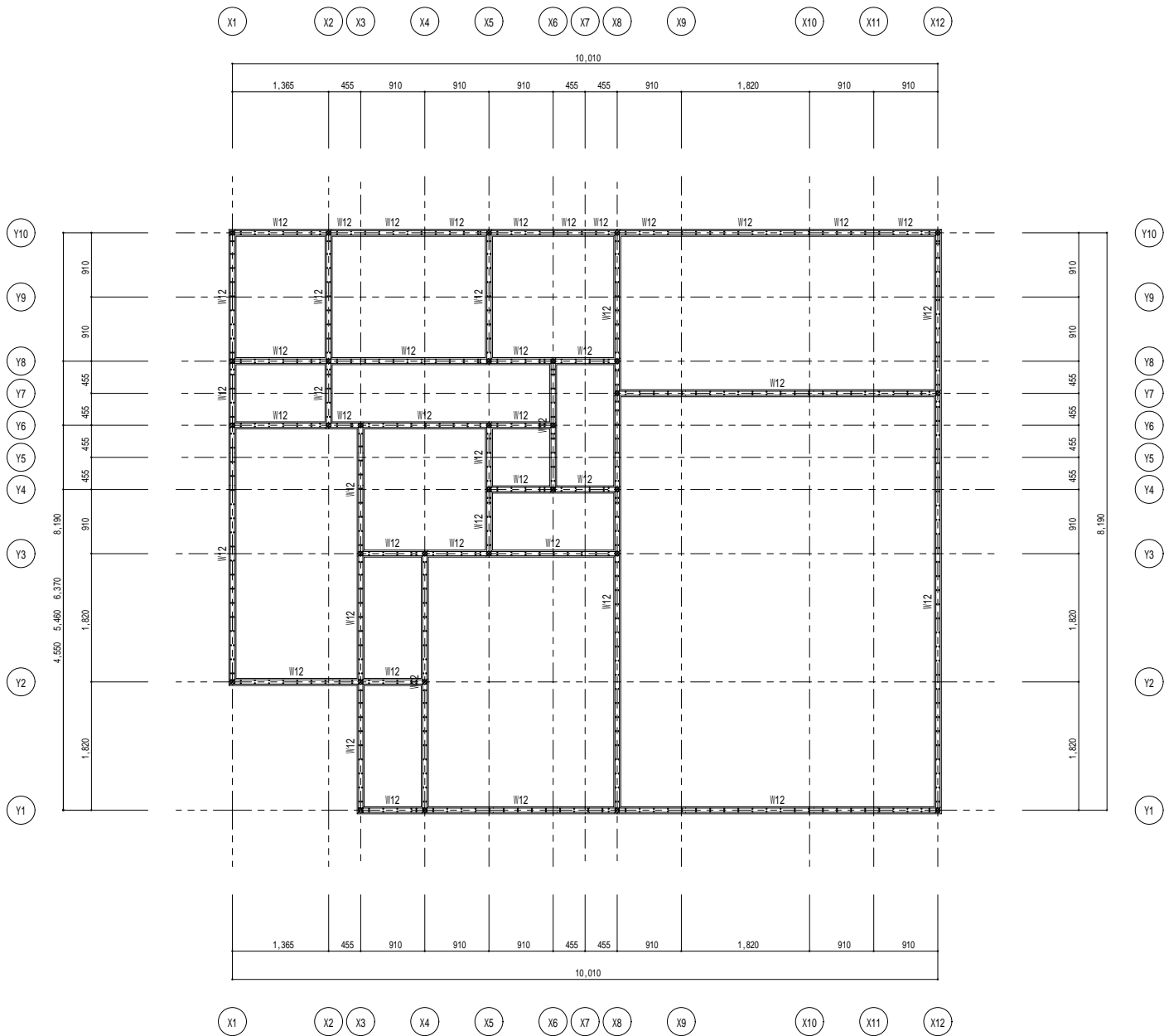
1 F 階平面詳細図 1 / 40
