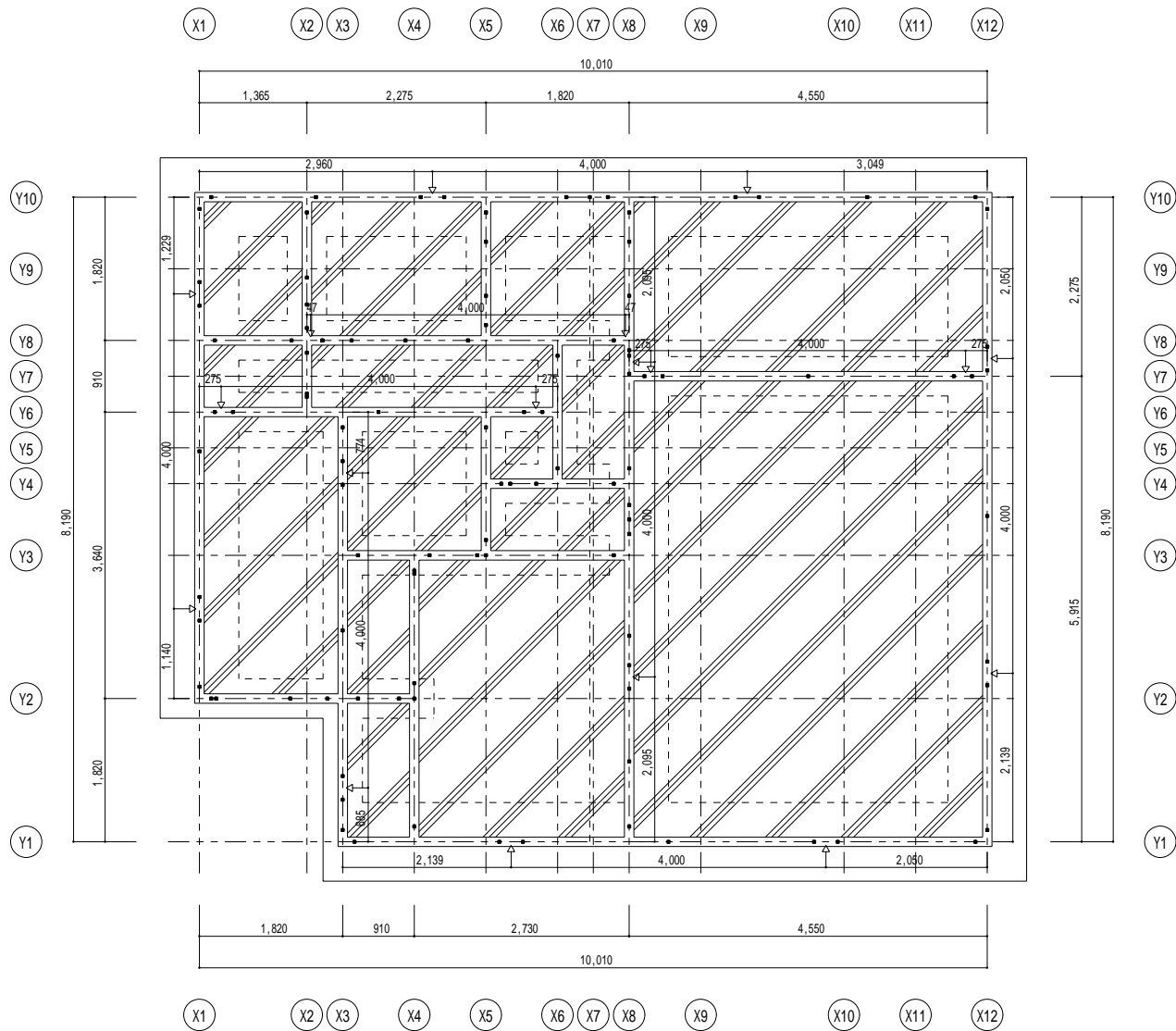
基础伏图 1/40
