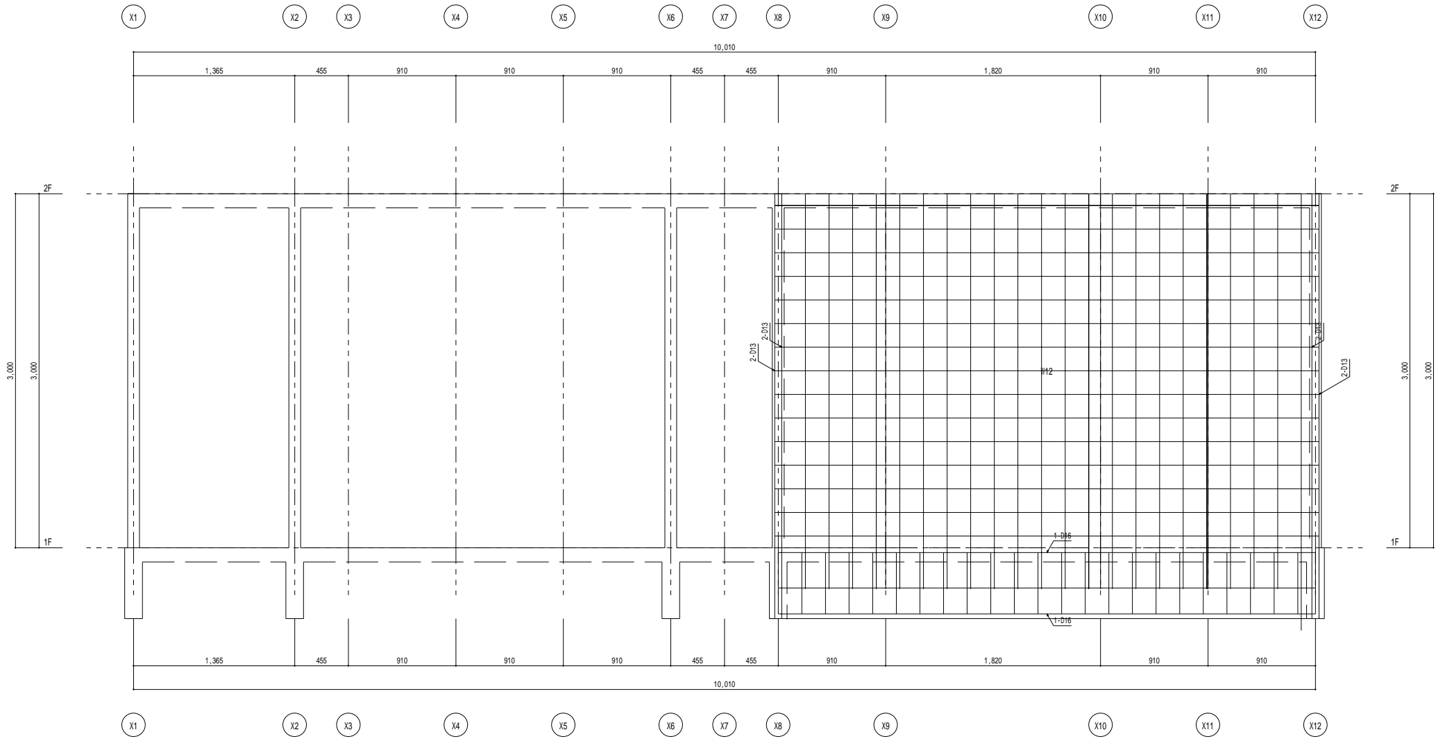
Y7通り架構詳細図 1 / 20
