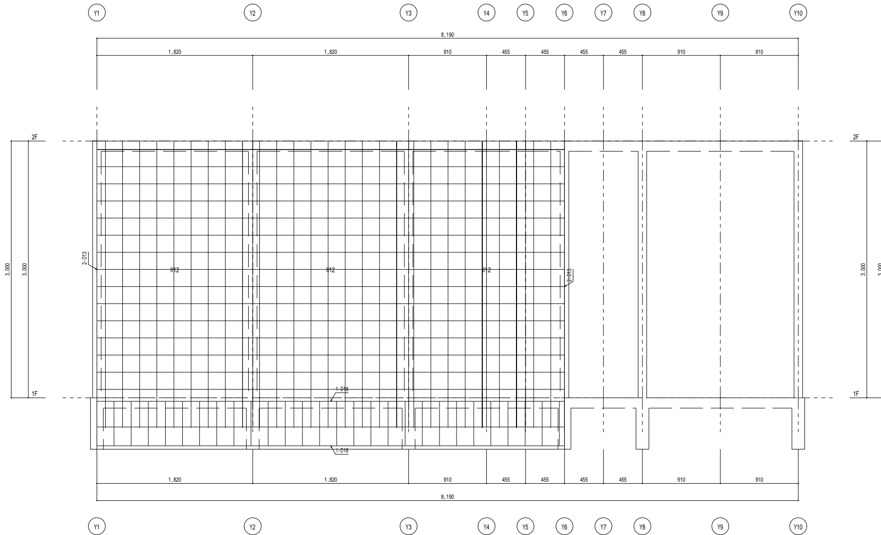
X 3 通り 架構 詳細図 1 / 2 0
