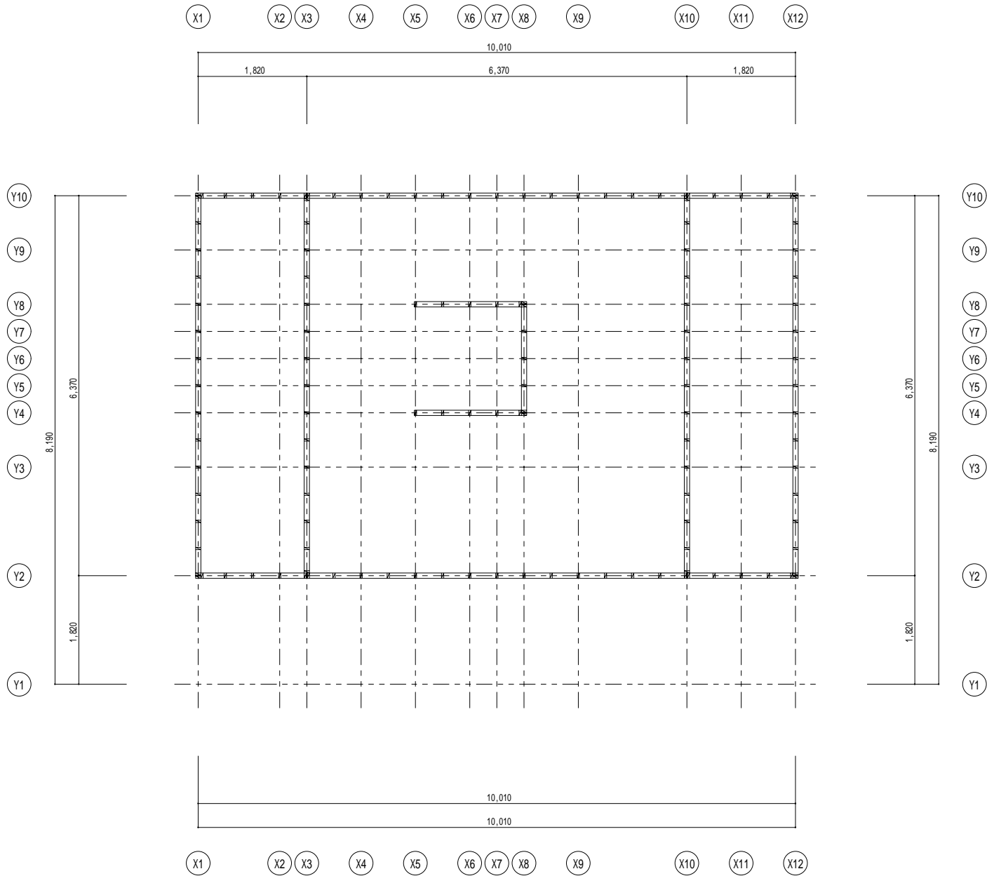
3F階たて枠伏図 1/40
