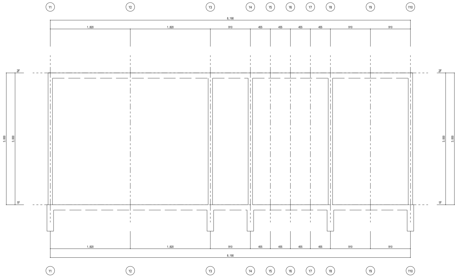
X 7 通り 架構 詳細 図 1 / 2 0
