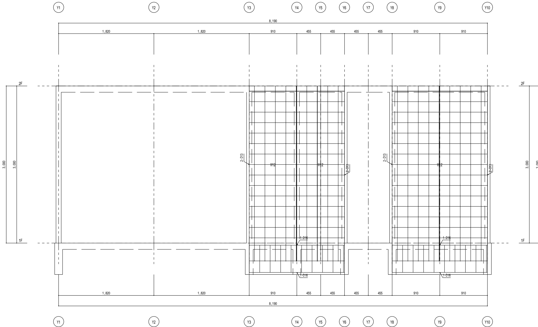
X 5 通り 架構 詳細 図 1 / 2 0
