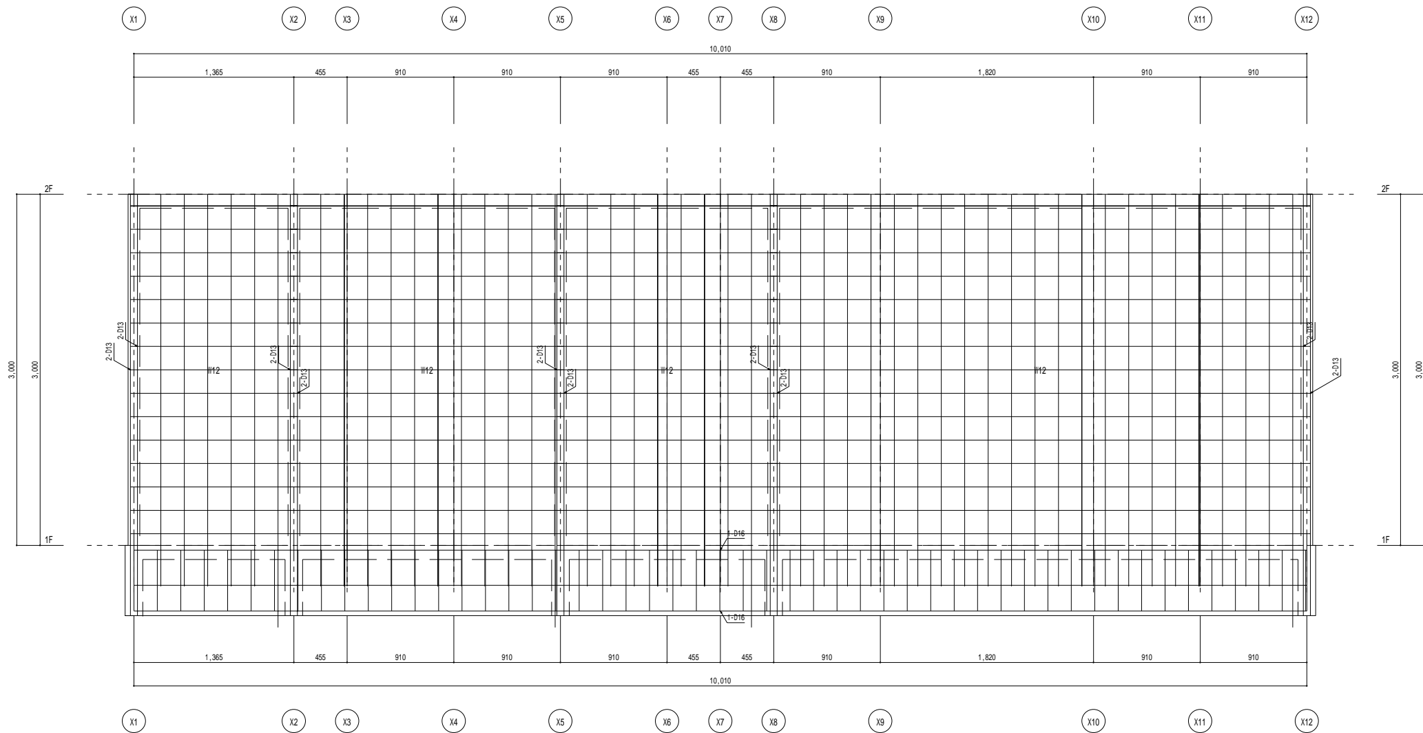
Y10 通り架構詳細図 1 / 2.0
