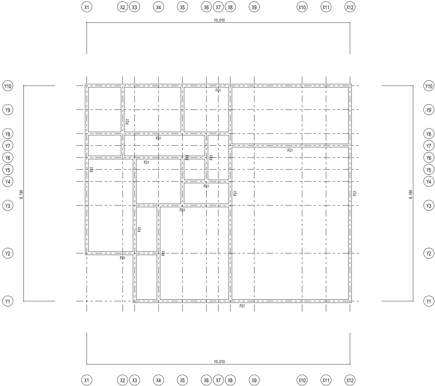
F階伏図 1/40
