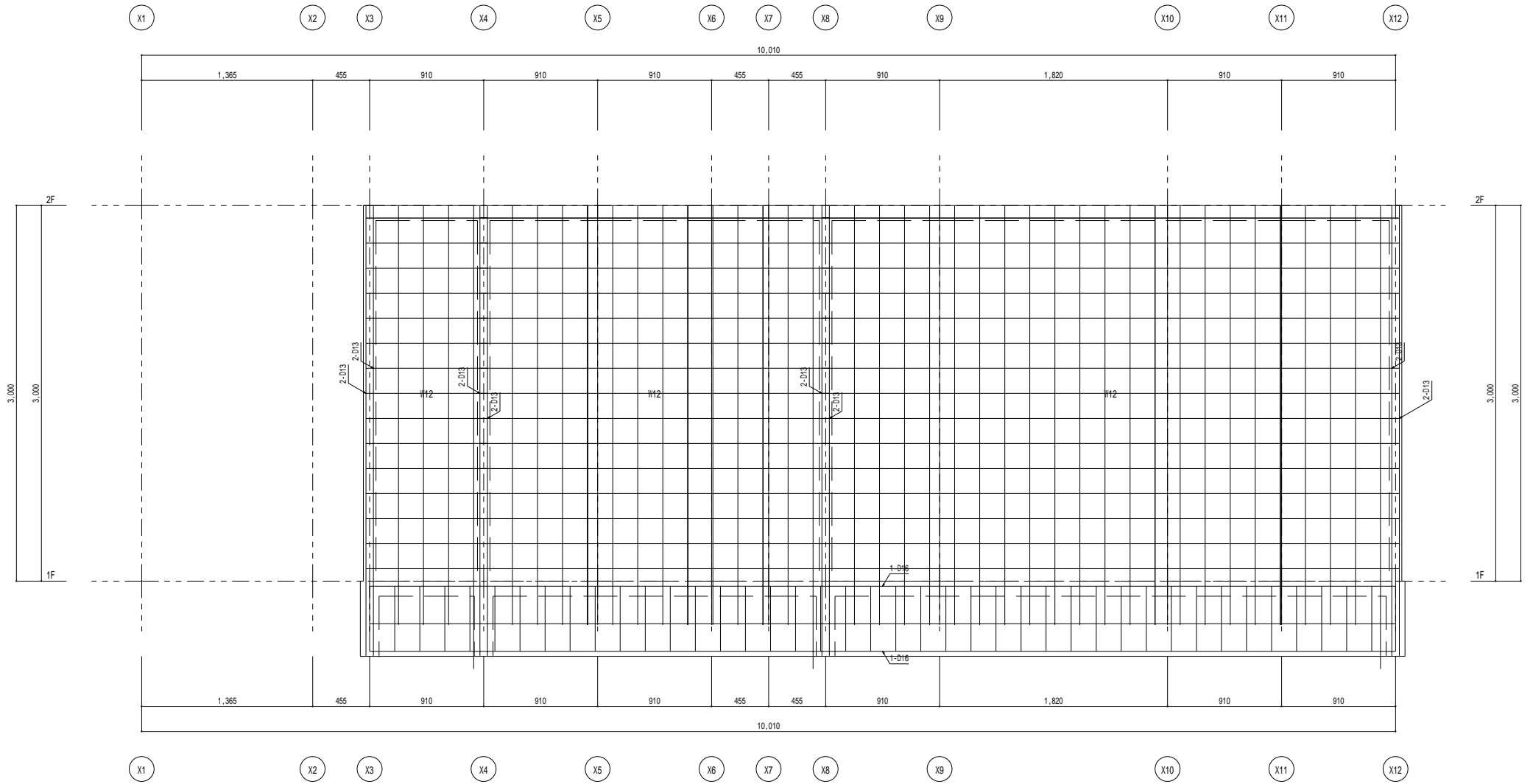
Y 1 通り架構詳細図 1 / 2 0
