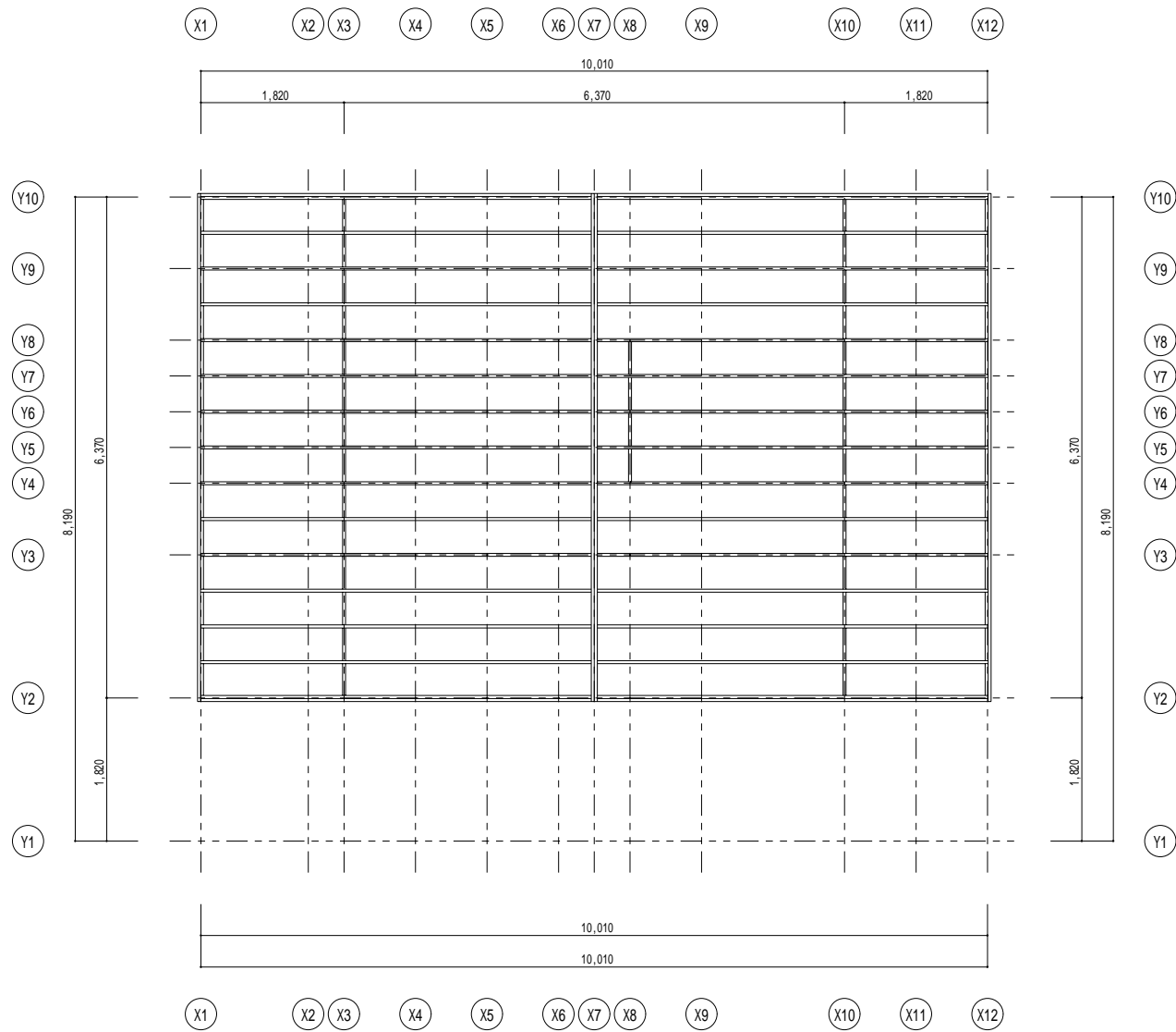
3F階床伏図 1/40
