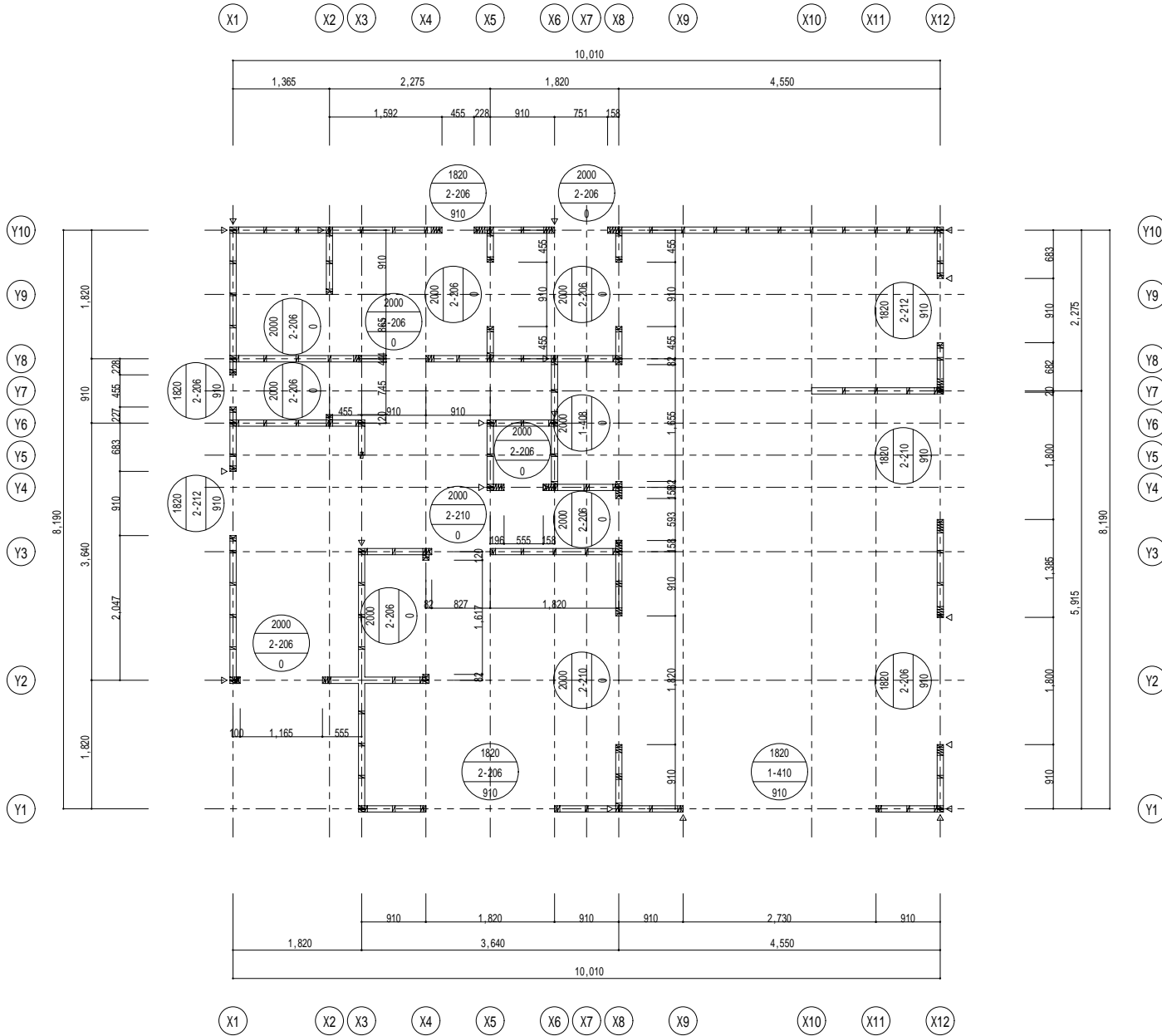
1F階たて枠伏図 1/40
