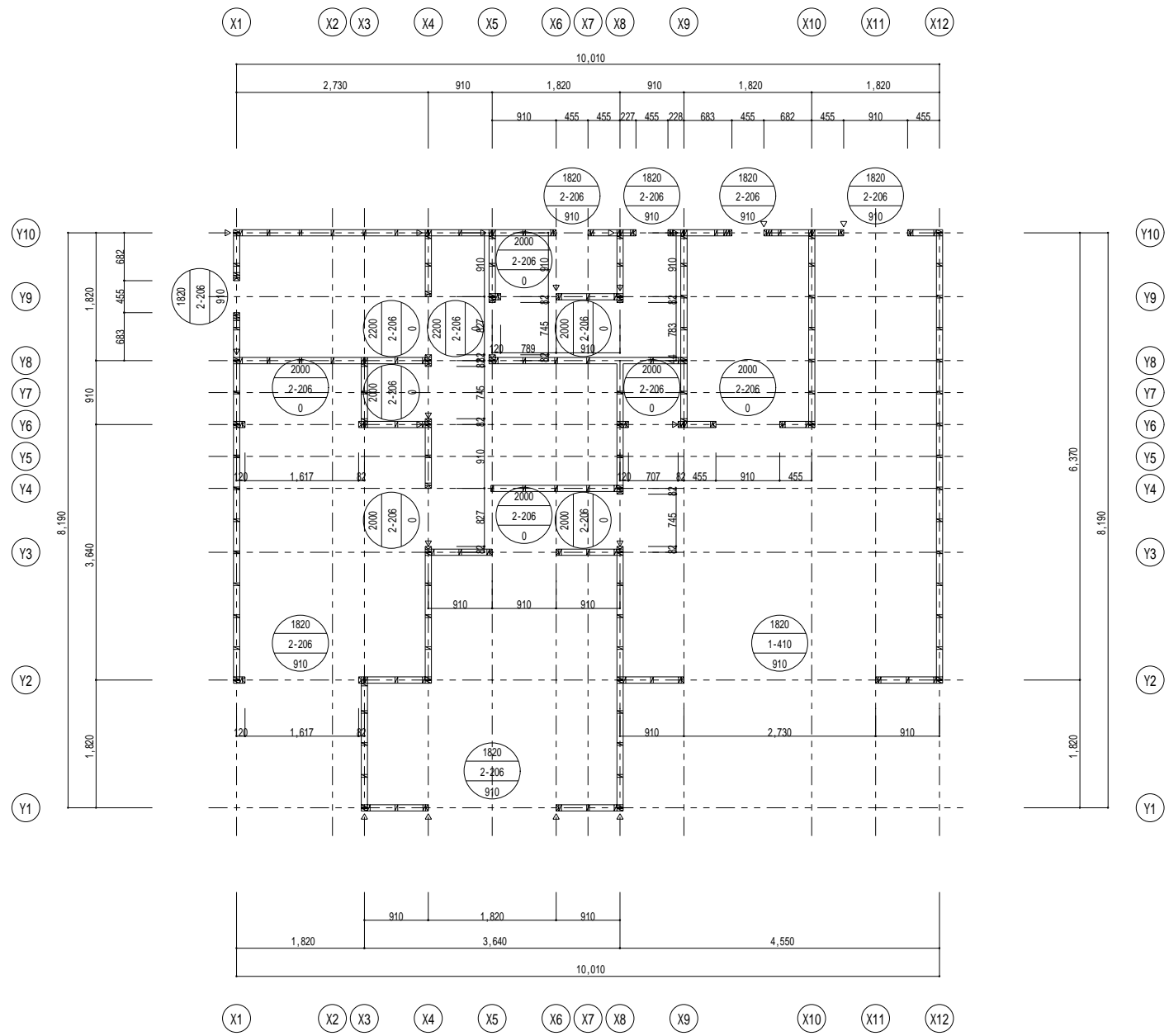
2F階たて枠伏図 1/40
