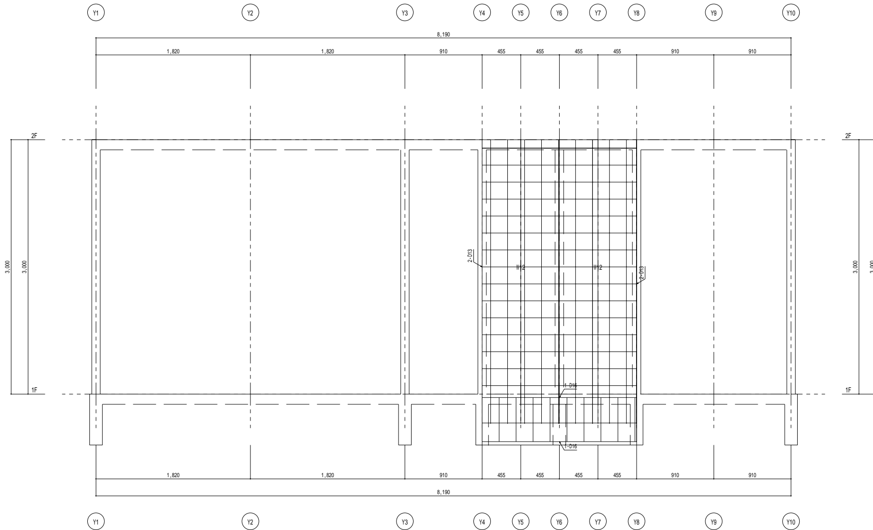
X 6 通り 架構詳細図 1 / 2 0
