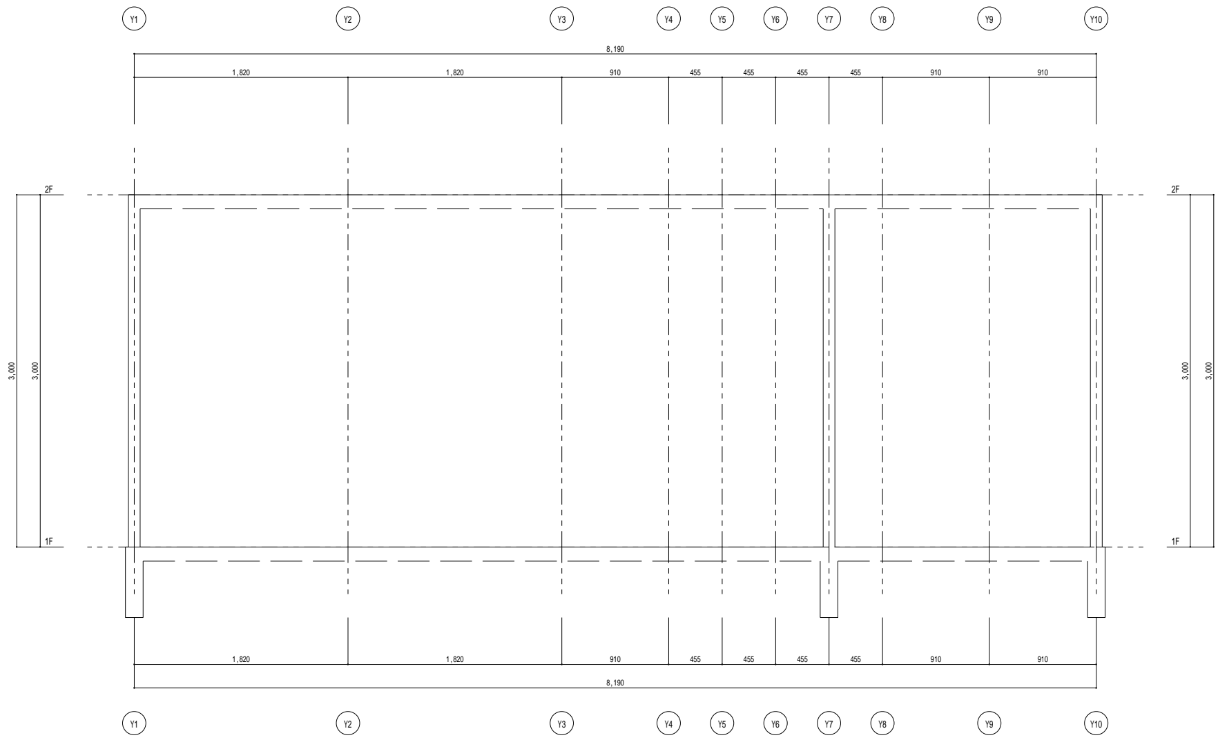
X 9 通り 架構 詳細図 1 / 2 0
