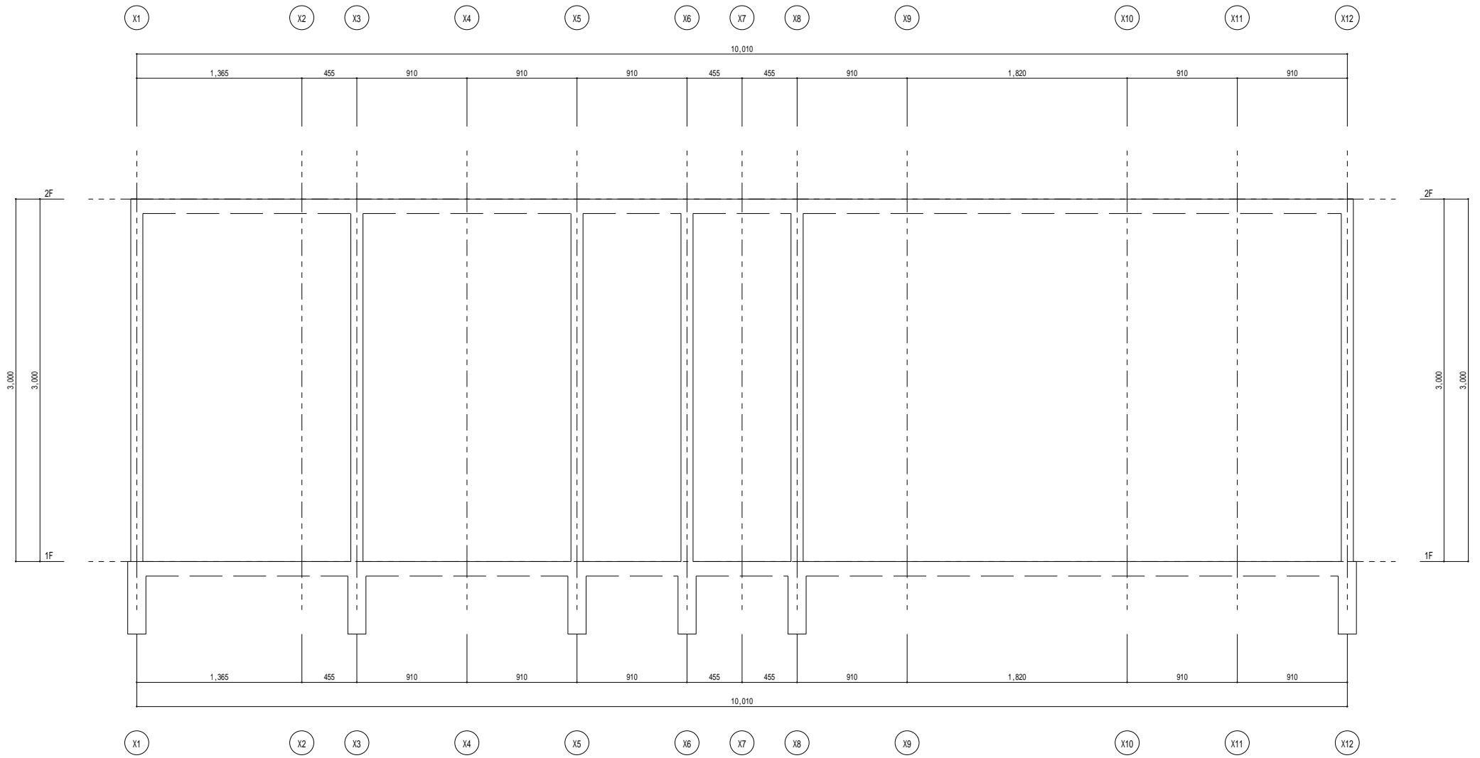
Y5通り架構詳細図 1 / 20
