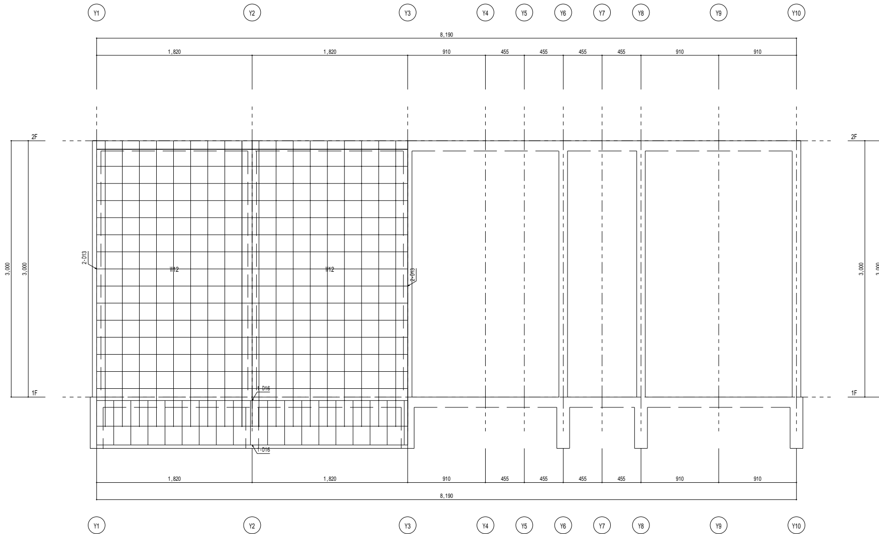
X 4 通り 架構 詳細 図 1 / 2 0
