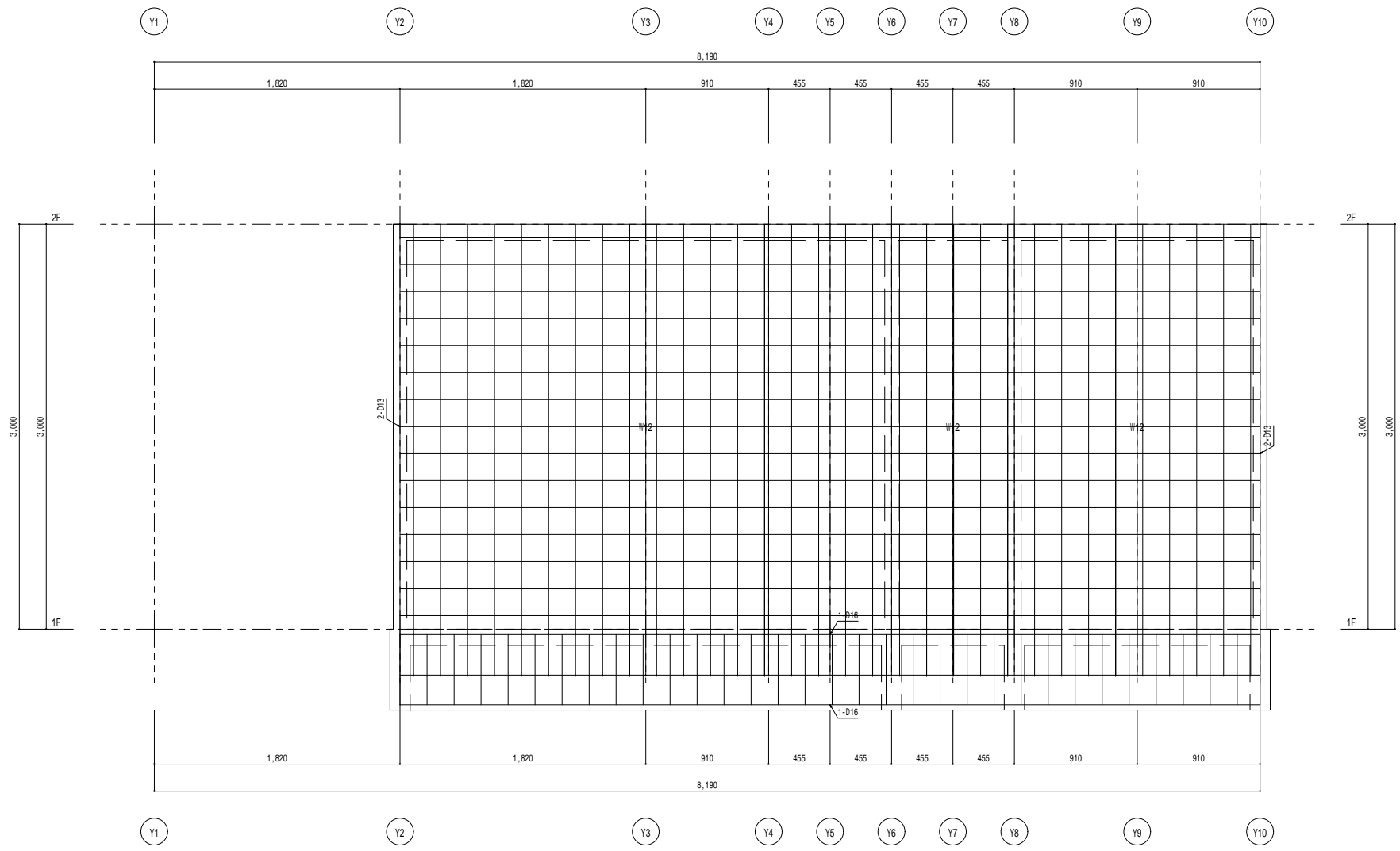
X 1 通り 架構 詳細図 1 / 2 0
