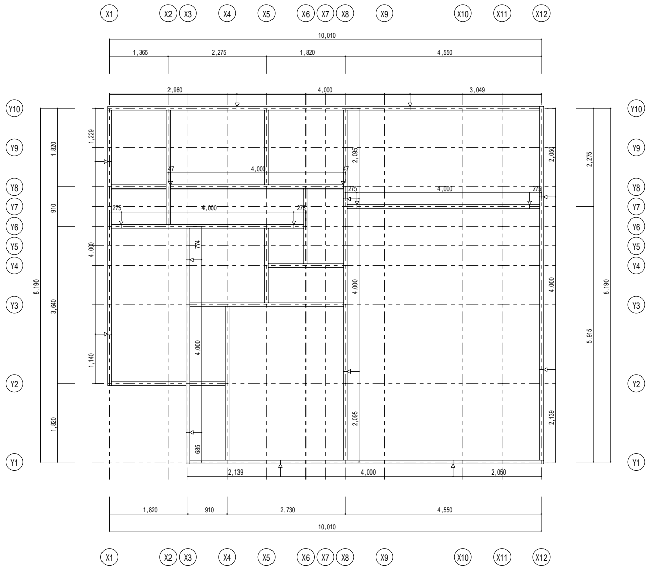
土台伏图 1/40
