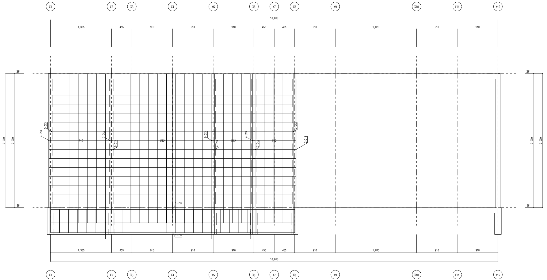
Y 8 通り架構詳細図 1 / 2 0
