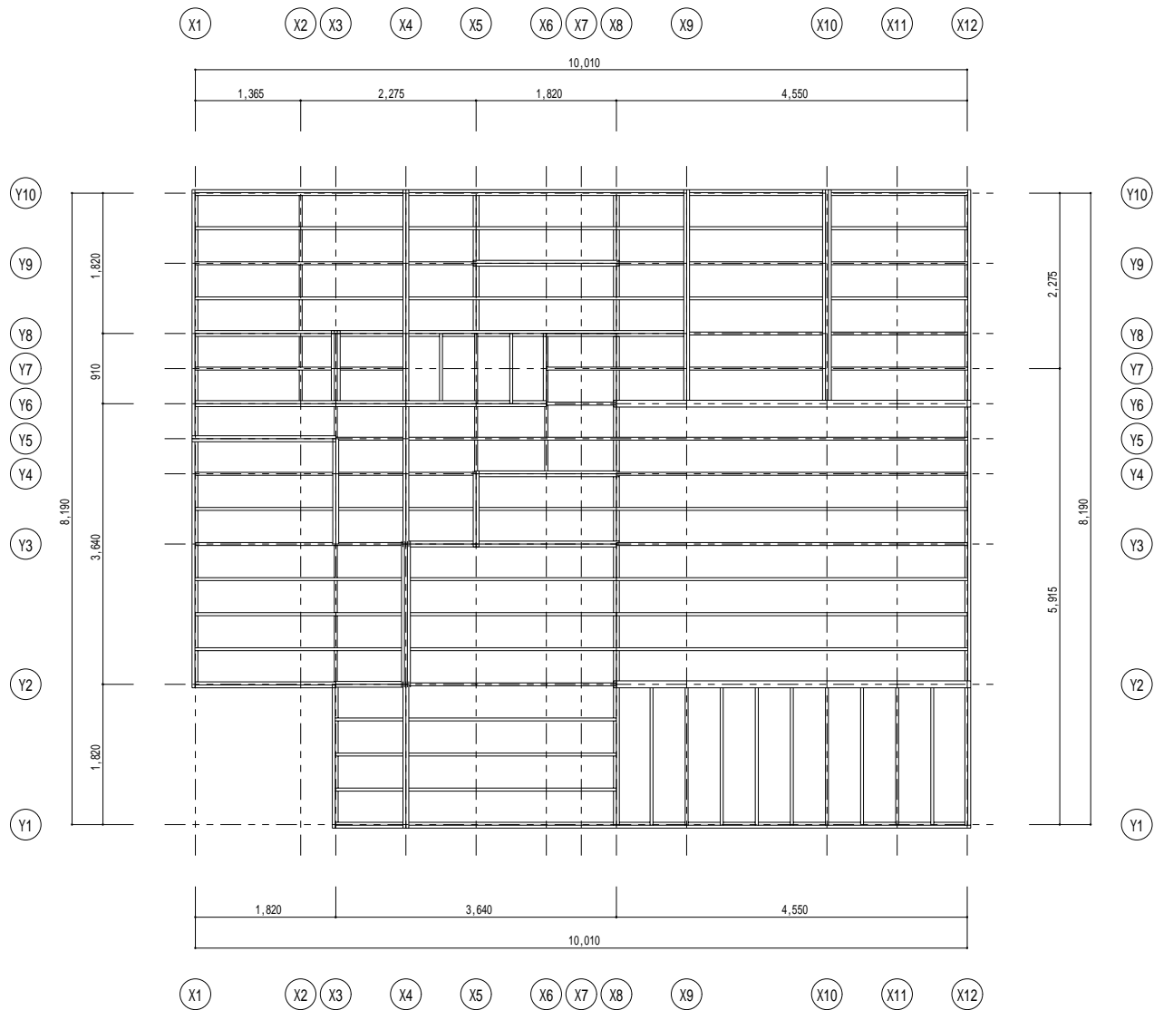
1F階床伏図 1/40
